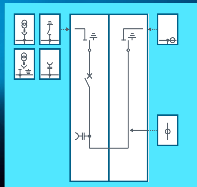
母线分段柜 BS
