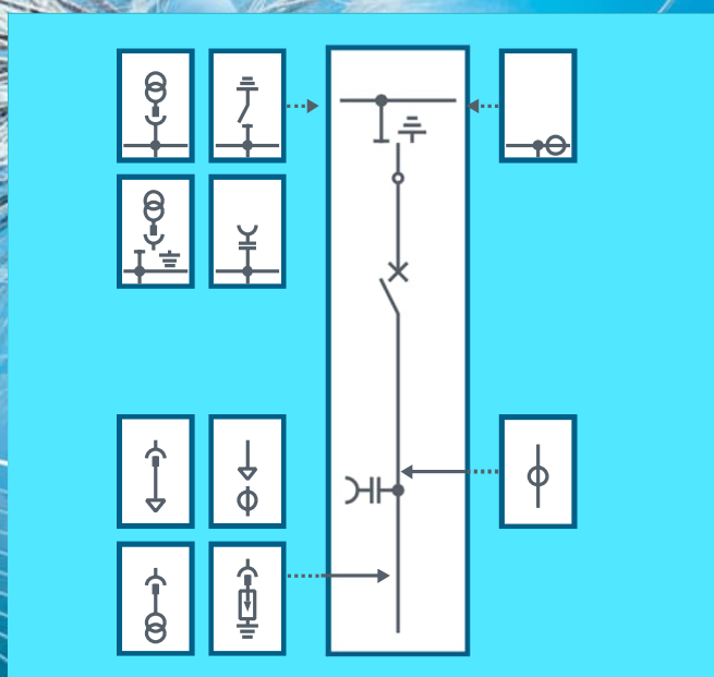
断路器柜 CB
