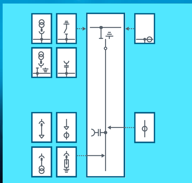
隔离开关柜 DS
