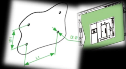
整体表面安装，前面板开孔
