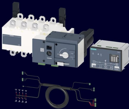
3KC7
