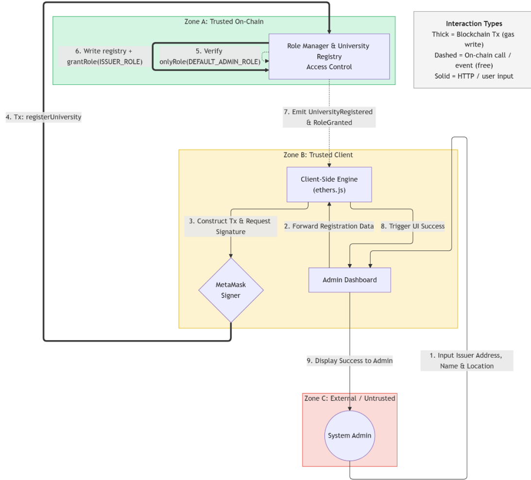
صورة 10 - تدفق تسجيل مؤسسة تعليمية ومنح دور الإصدار
