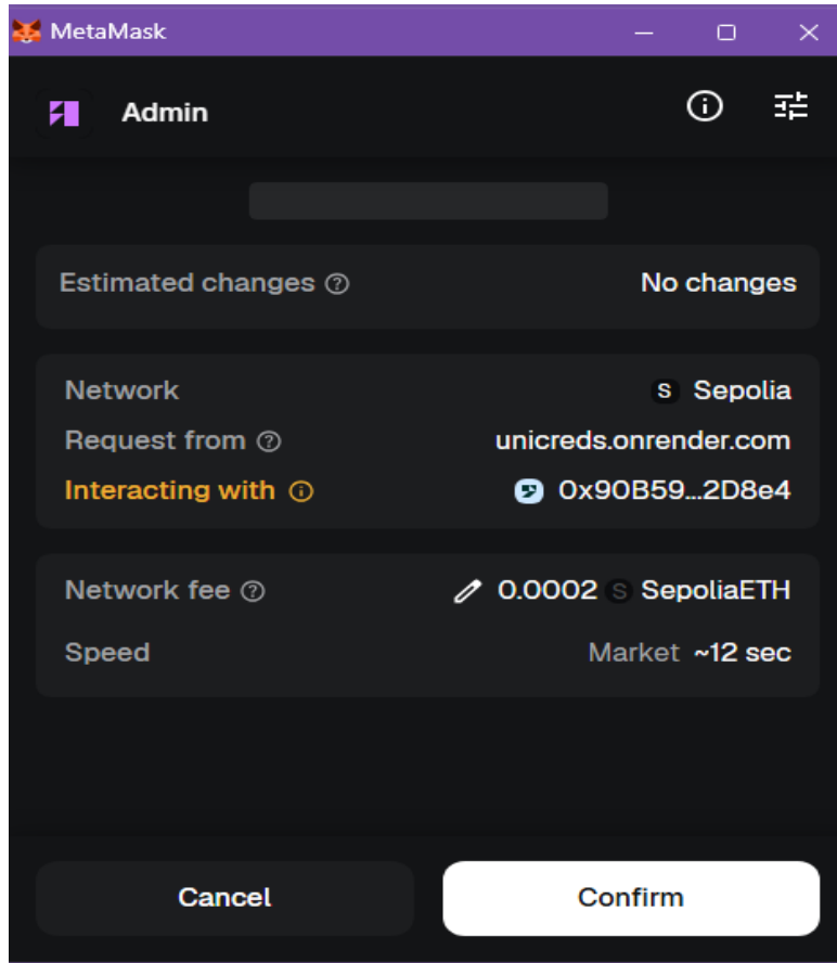
صورة 24 - نافذة MetaMask لتأكيد معاملة تنشيط جامعة موقوفة مسبقاً
