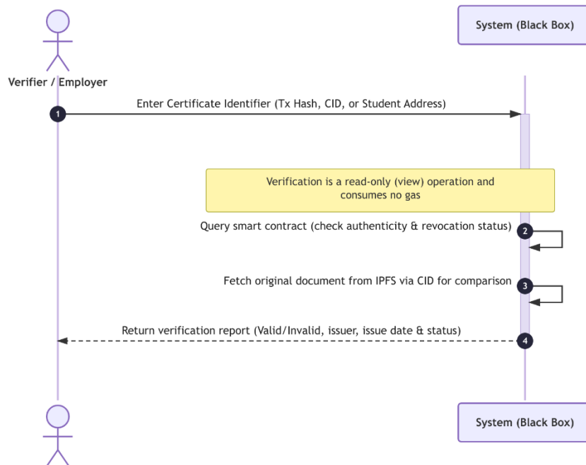
صورة 5 - مخطط تسلسل النظام - التحقق من صحة ومصدر الشهادة
