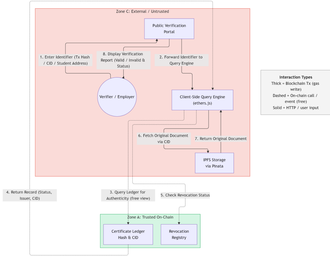
صورة 13 - تدفق التحقق من صحة الشهادة
