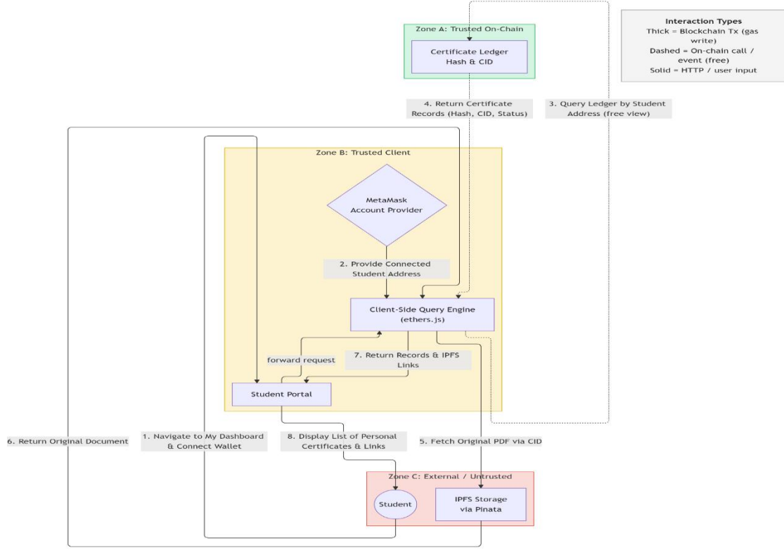
صورة 14 - تدفق استعراض الطالب لشهاداته
