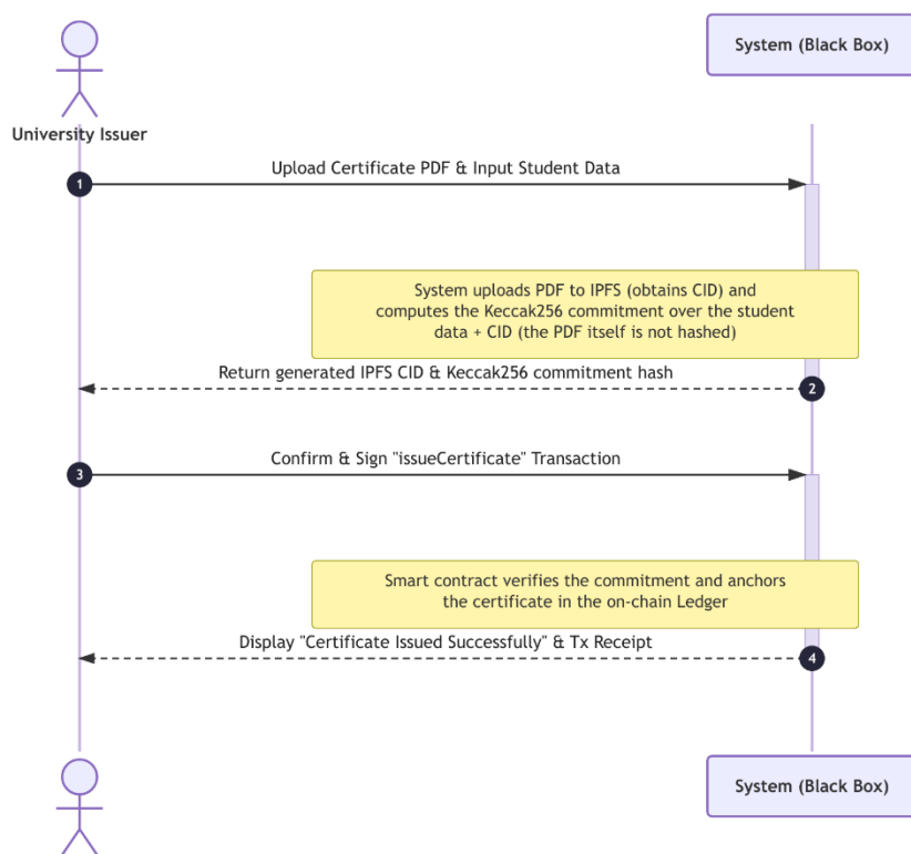
صورة 3 - مخطط تسلسل النظام - إصدار وتوثيق شهادة رقمية
