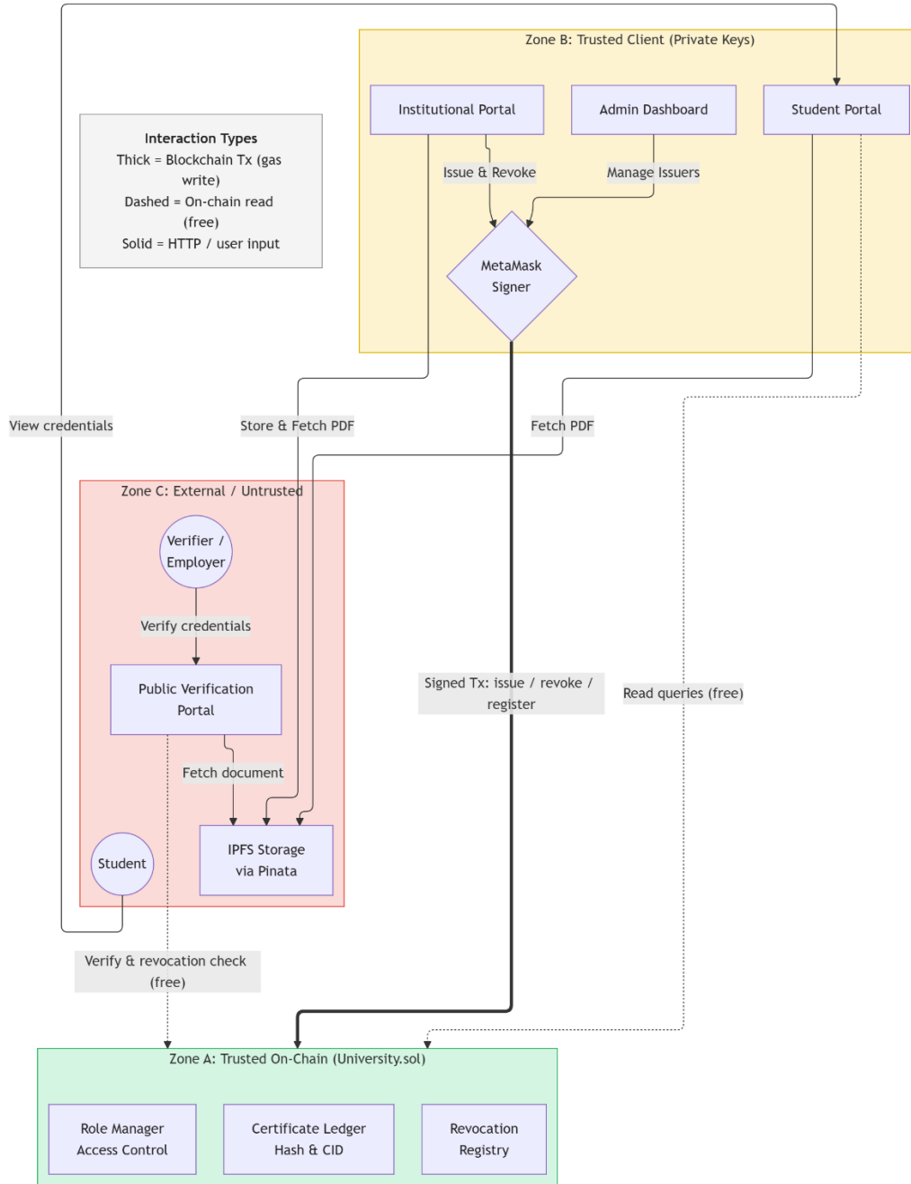
صورة 7 - المعمارية العامة للنظام وتوزع مناطق الثقة
