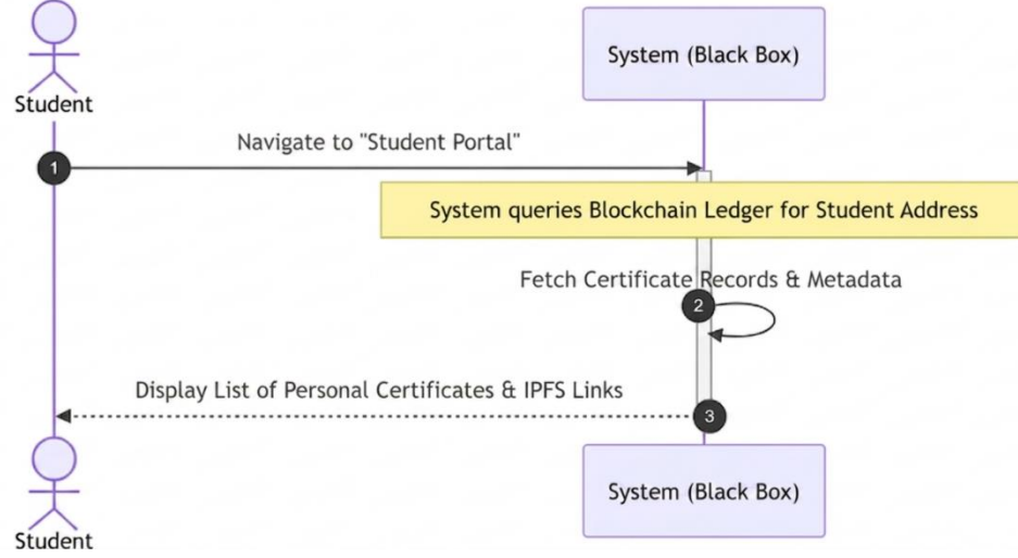
صورة 6 - مخطط تسلسل النظام - استعراض الطالب لسجله الأكاديمي والتحقق منه
