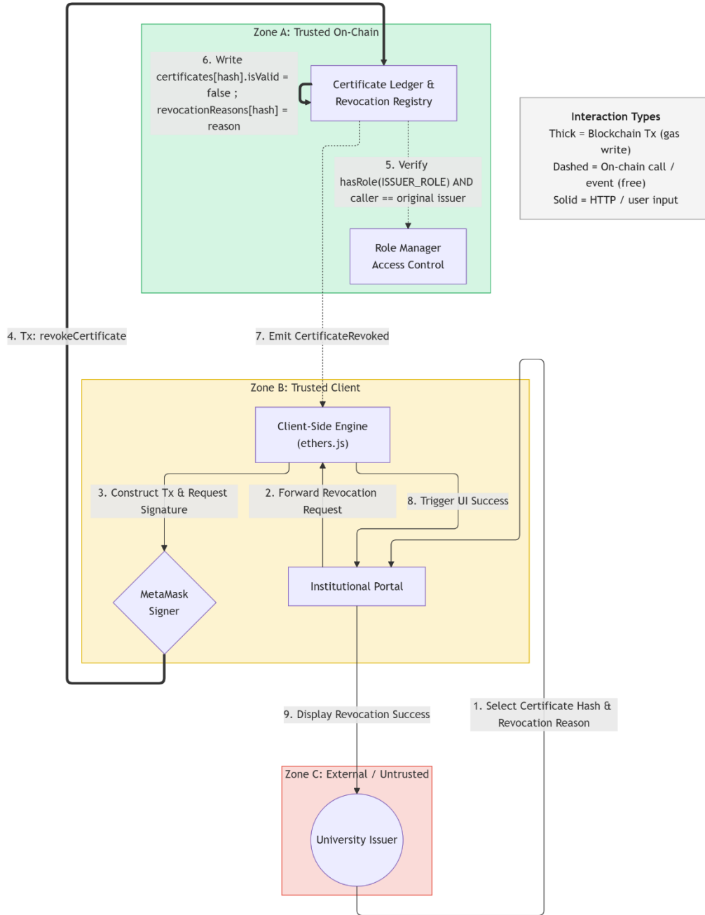
صورة 12 - تدفق إلغاء الشهادة
