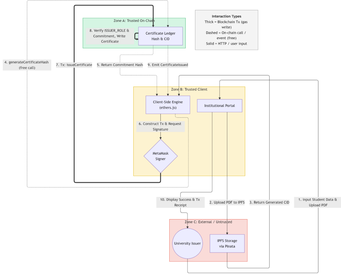
صورة 11 - تدفق إصدار شهادة
