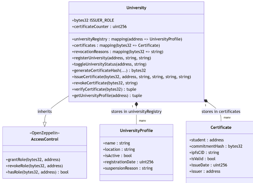
صورة 8 - مخطط الأصناف (Class Diagram) للعقد الذكي University.sol
