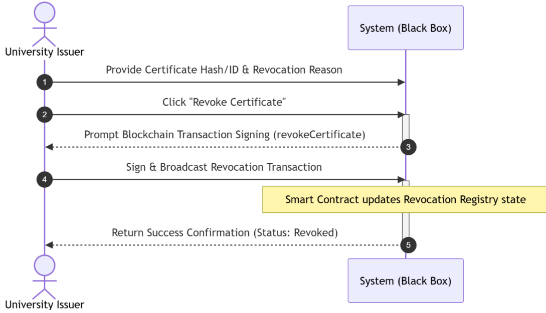
صورة 4 - مخطط تسلسل النظام - إلغاء شهادة صادرة
