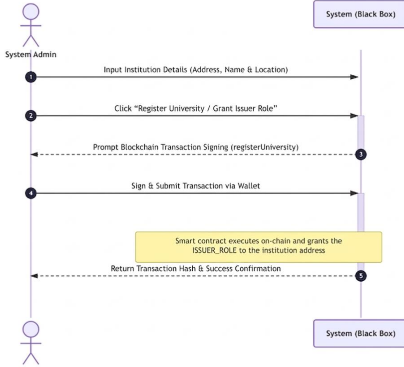
صورة 2 - مخطط تسلسل النظام - تسجيل مؤسسة أكاديمية وتفويضها
