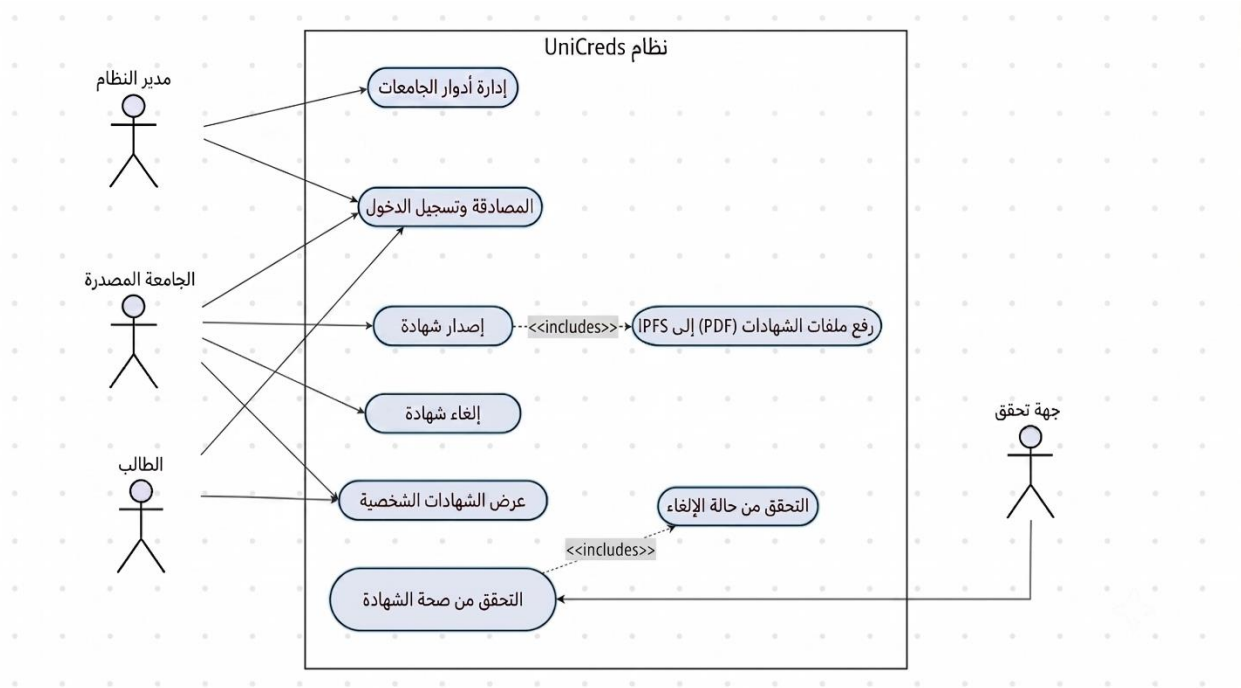
صورة 1 - مخطط حالات الاستخدام لنظام UniCreds
