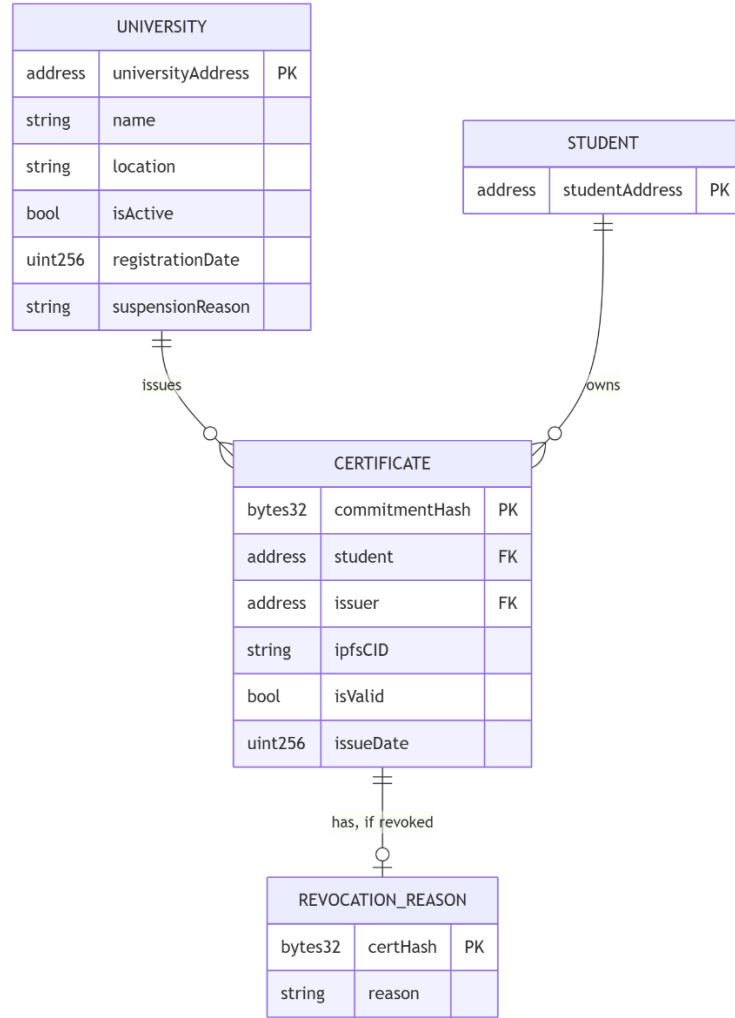
صورة 9- مخطط العلاقات بين هياكل البيانات المخزنة على السلسلة (بديل عن ERD نظراً لعدم وجود قاعدة بيانات علائقية)
