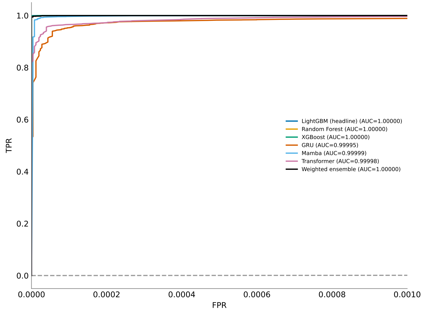
ROC (zoom: FPR \leq 1e-3 )
