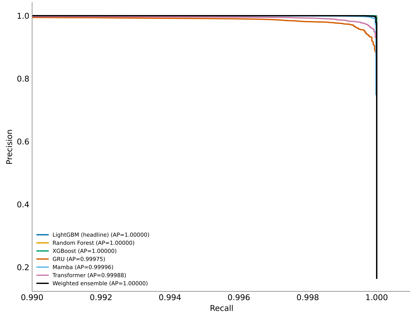
Precision-Recall (zoom)
