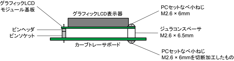
グラフィックLCDモジュールの組み立て状態
