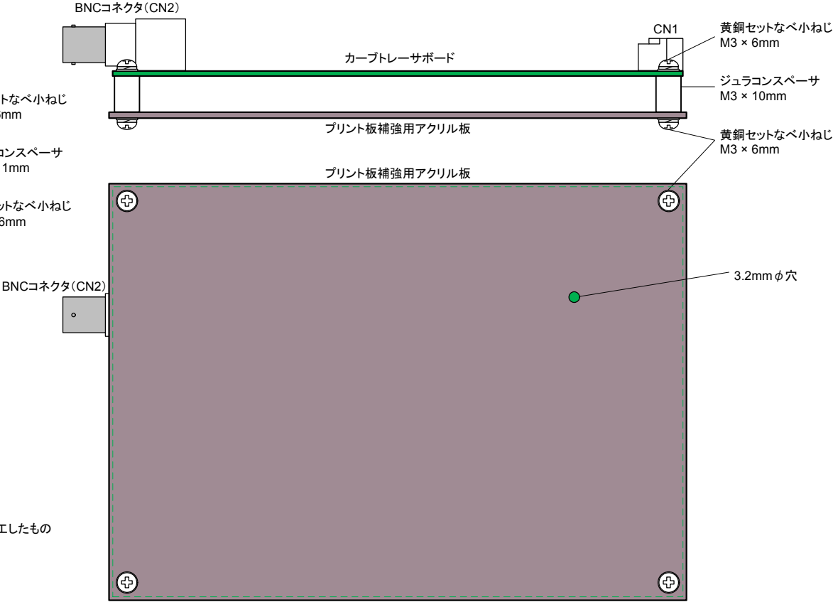
プリント板補強用アクリル板の組み立て状態
