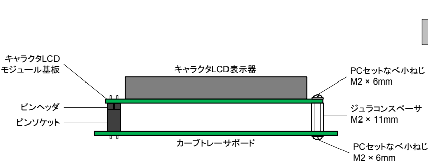
キャラクタLCDモジュールの組み立て状態
