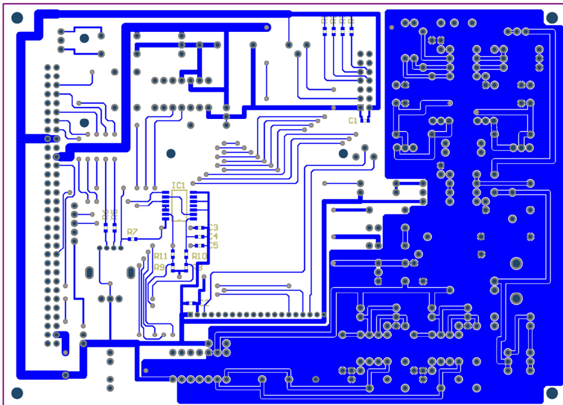
(b) はんだ面
