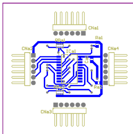
プリント板配線図
