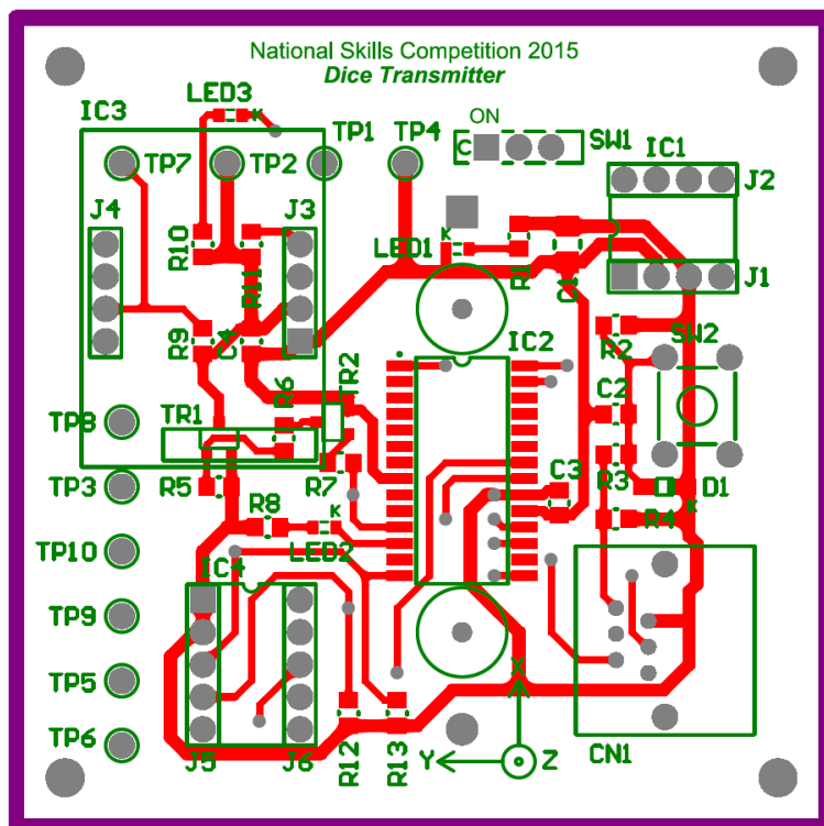
部品配置図
