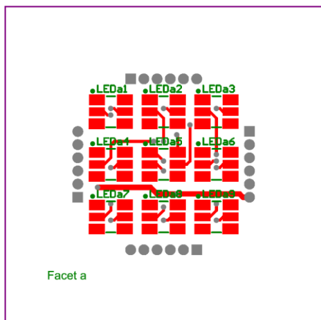
部品配置図
