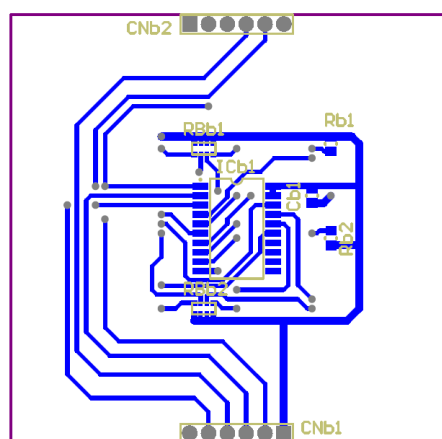
プリント基板配線図
