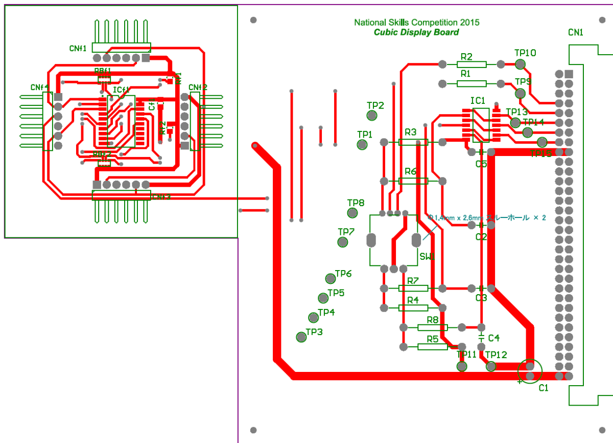
部品配置図
