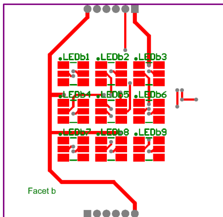
部品配置図
