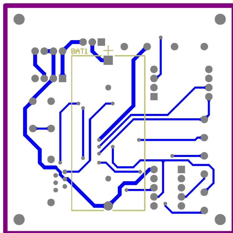
プリント板配線図
