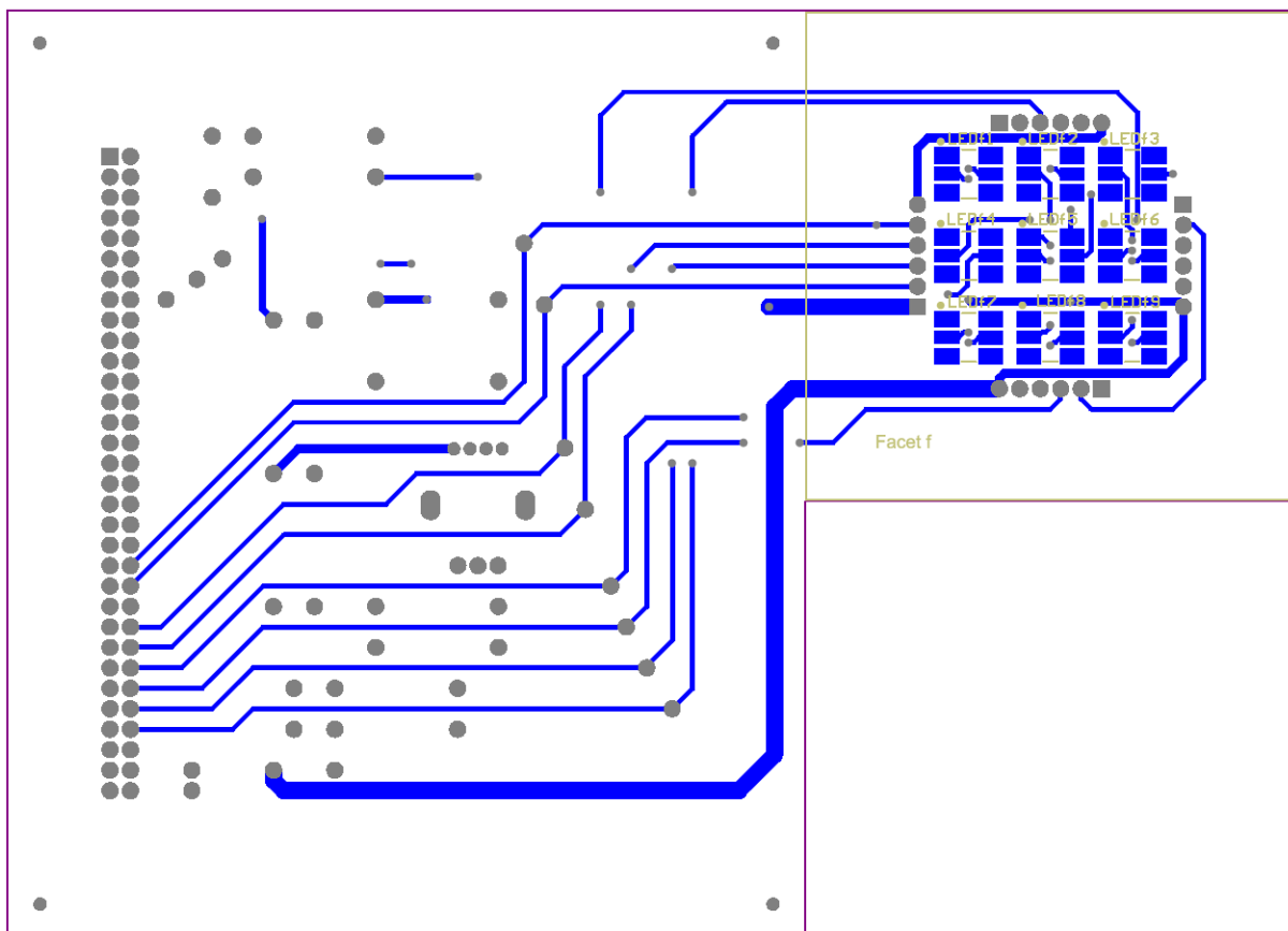
プリント板配線図
