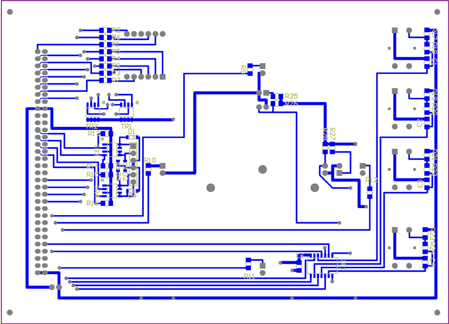
「クロックボード」基板図 B 面
