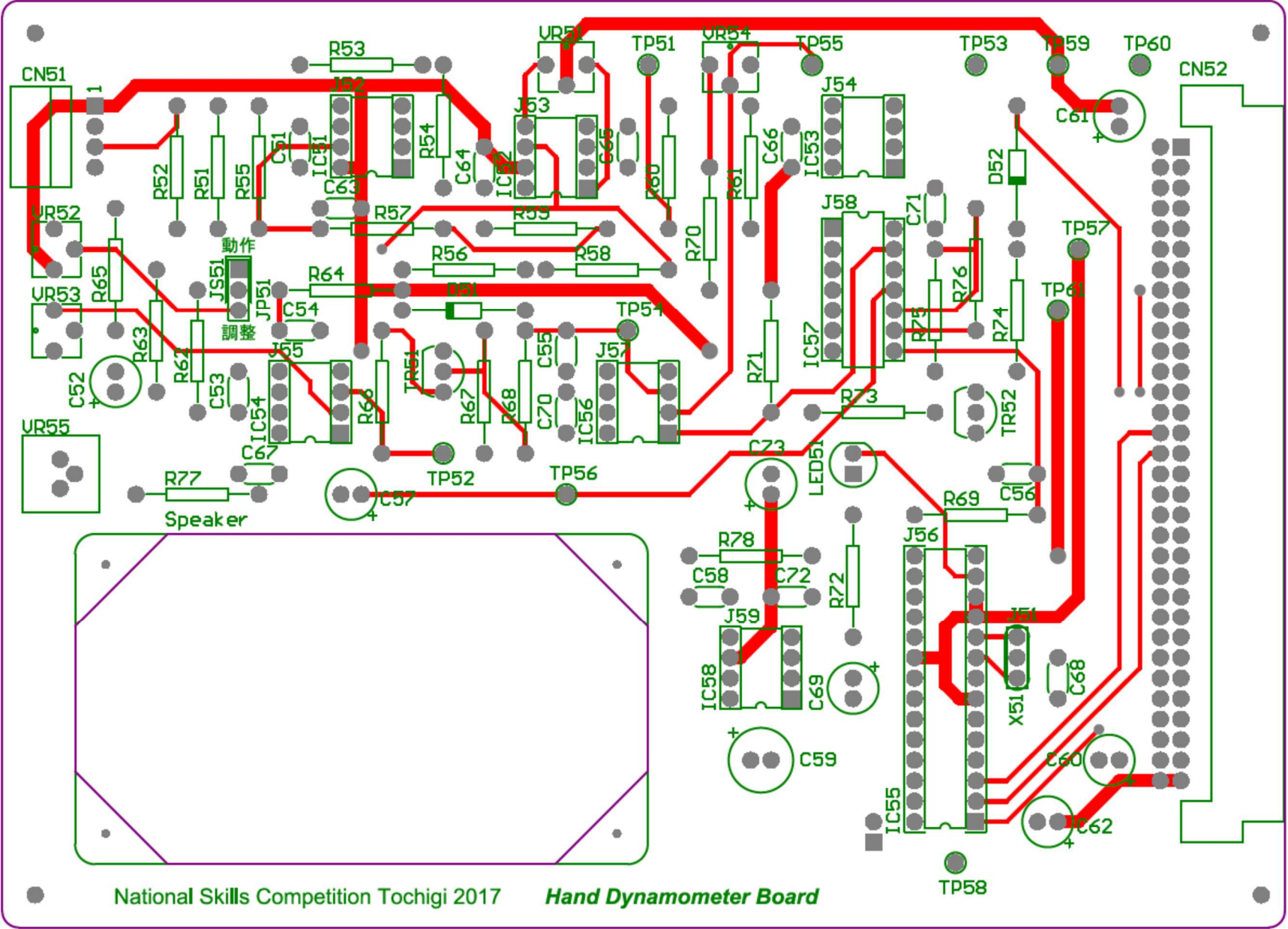
「握力計ボード」基板図 A 面
