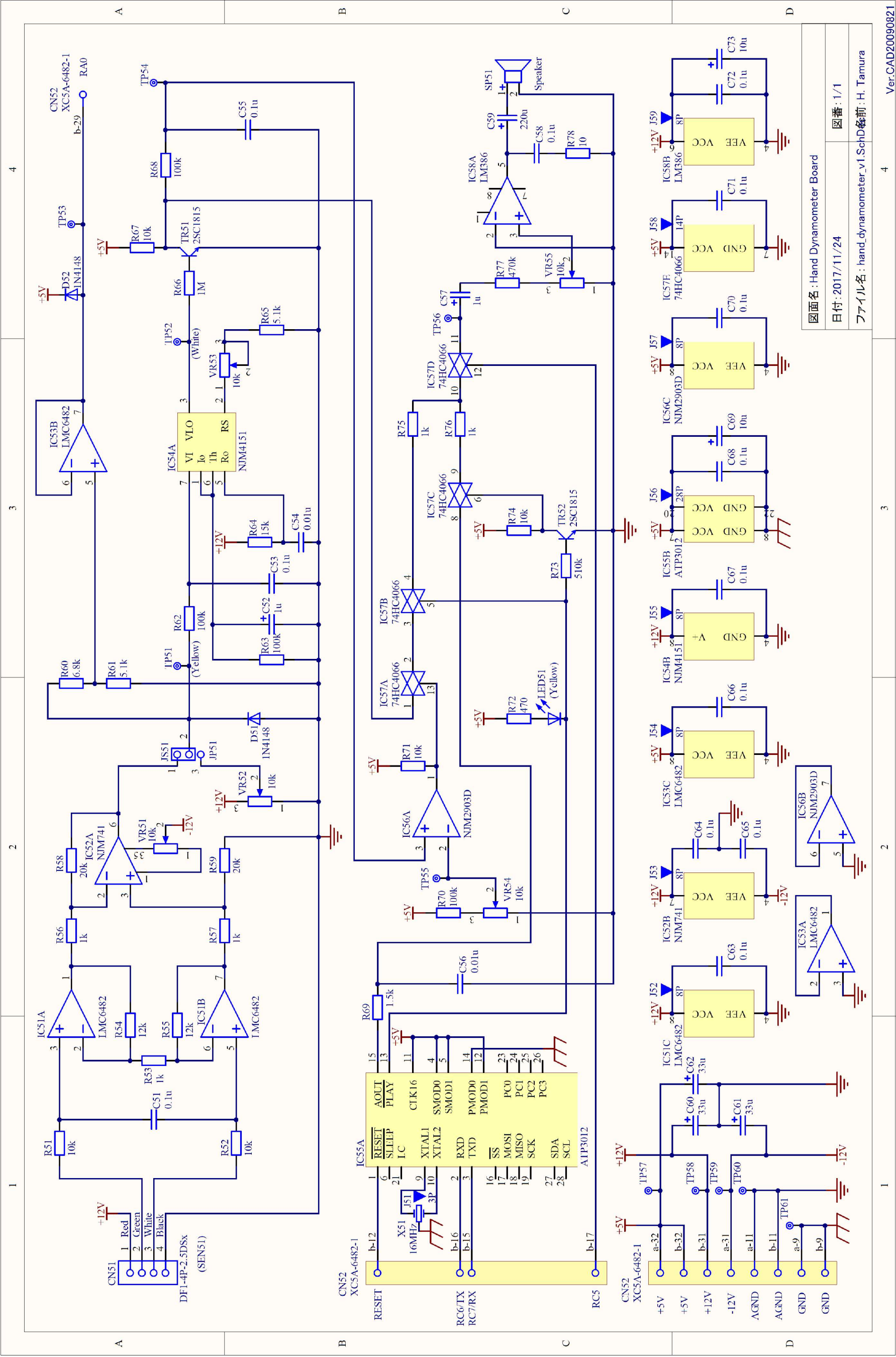
「握力計ボード」回路図
