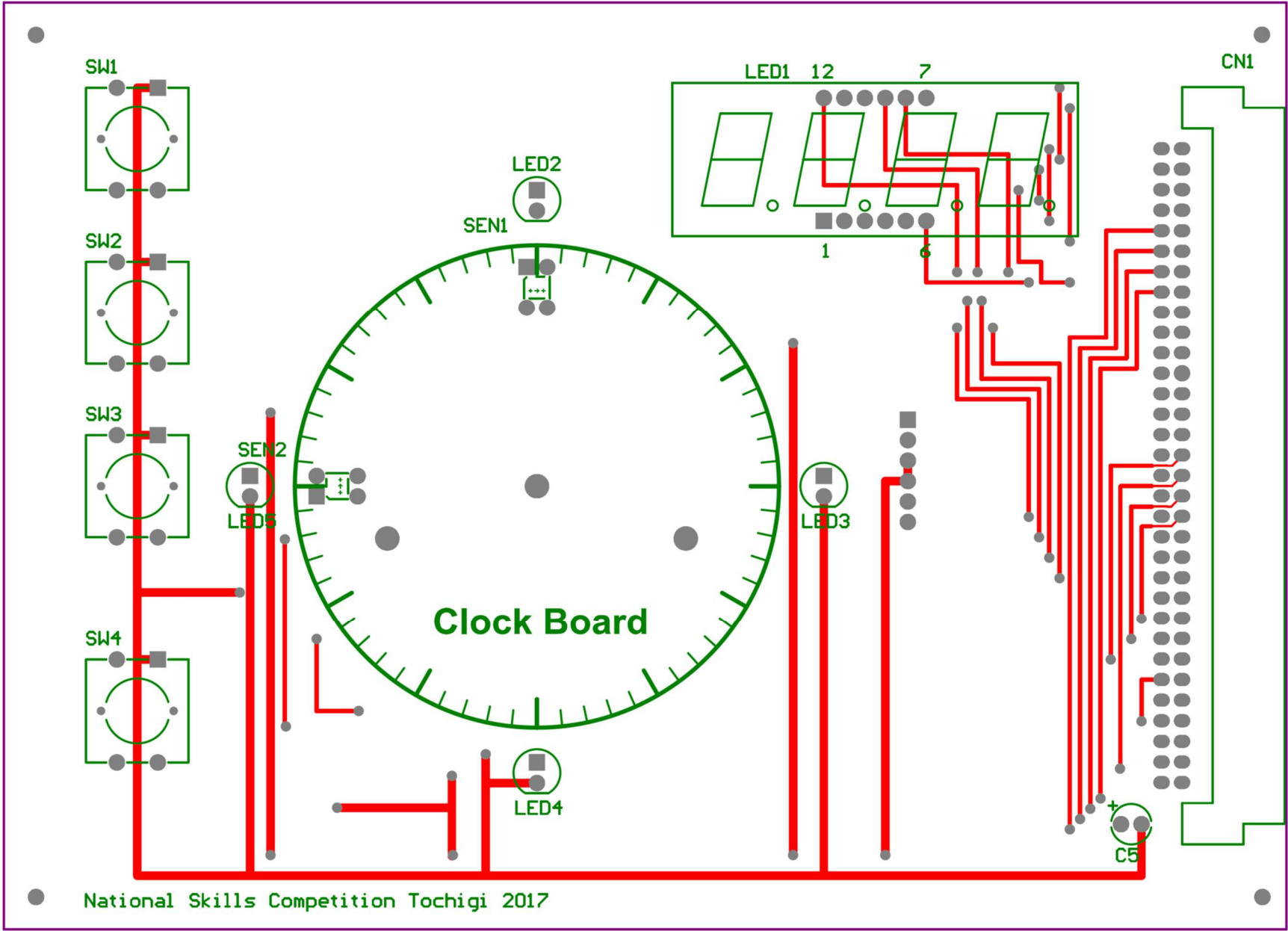
「クロックボード」基板図 A 面
