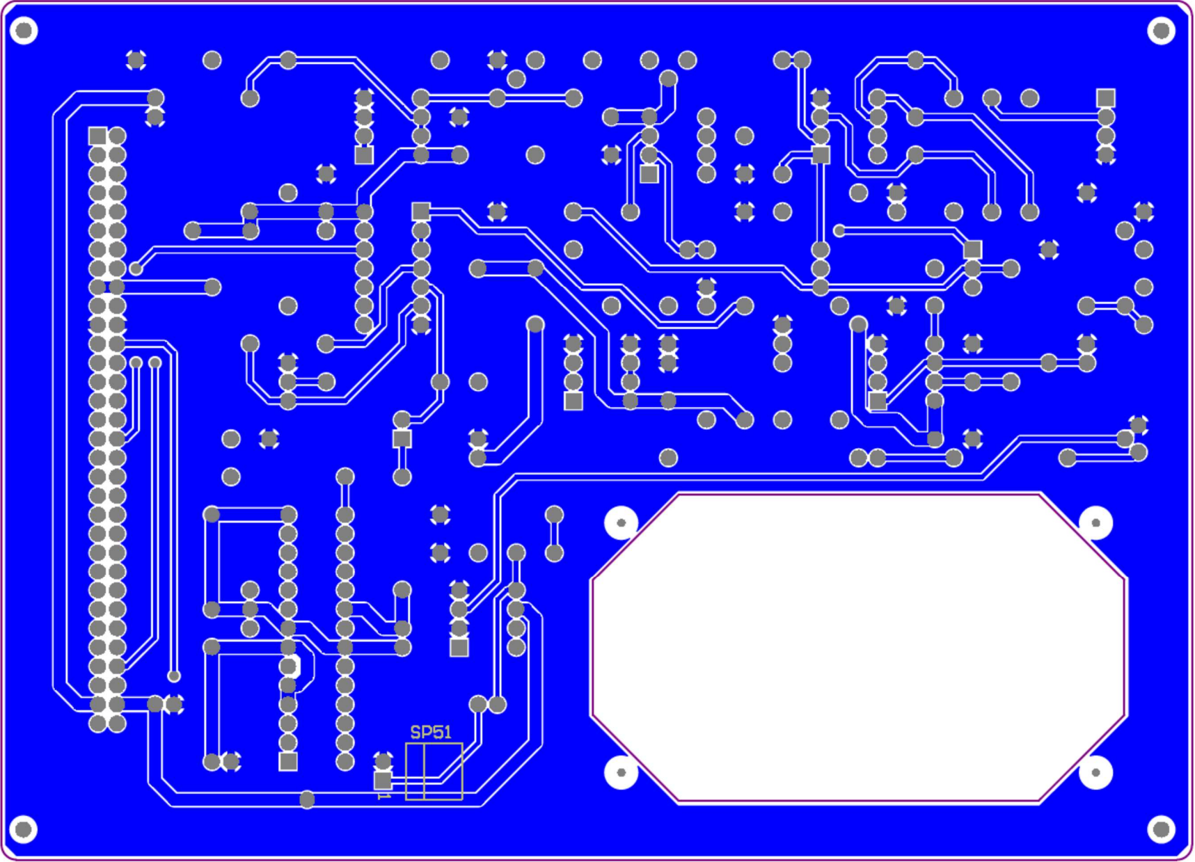
「握力計ボード」基板図 B 面
