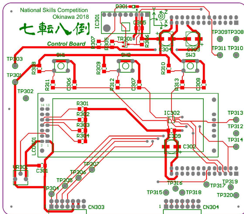
図 A3-8 「コントロールボード」基板図 A 面
