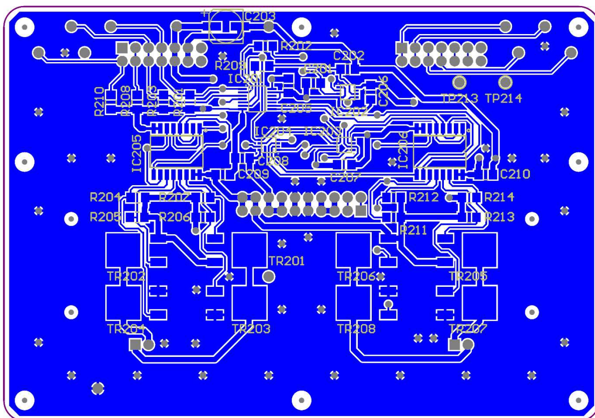
図 A3-7 「モータボード」 基板図 B 面
