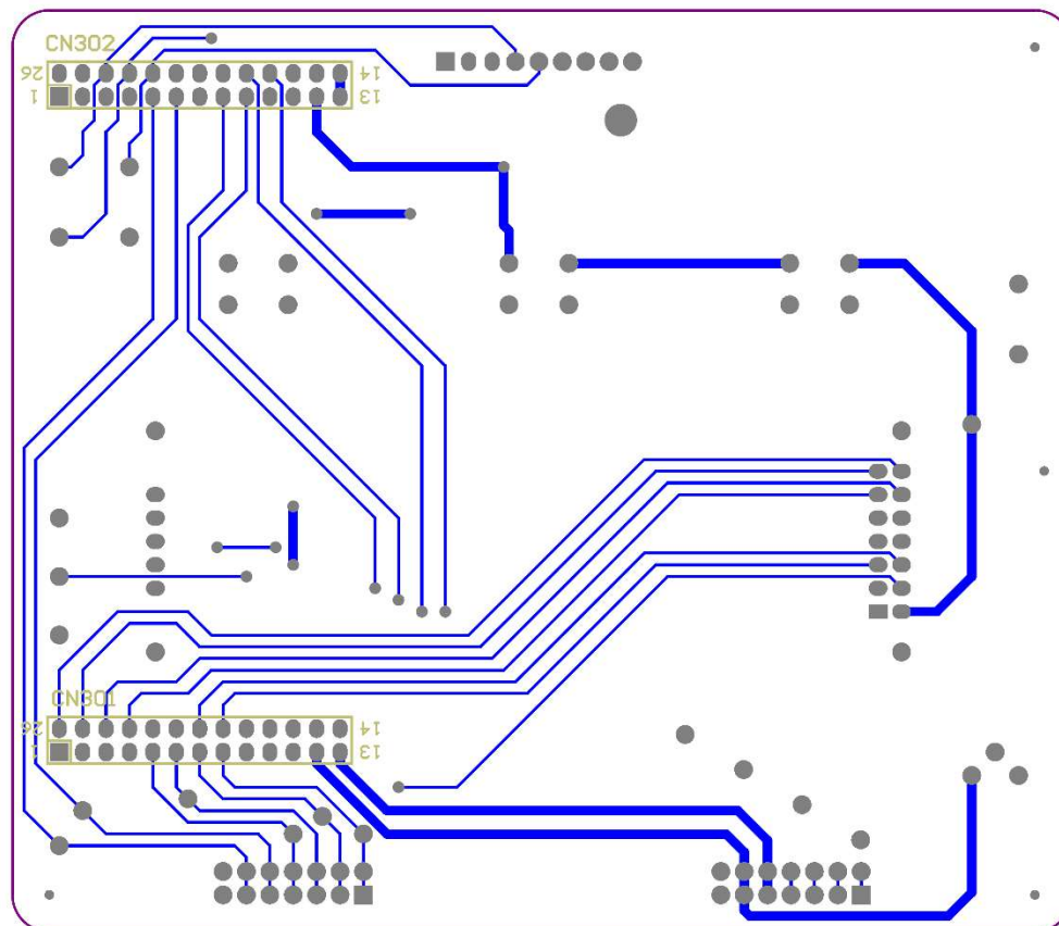
図 A3-9 「コントロールボード」基板図 B 面
