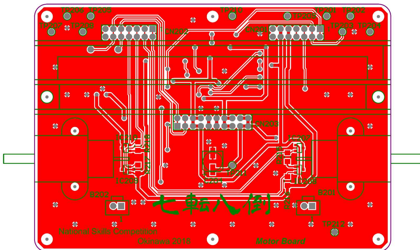
図 A3-6 「モータボード」 基板図 A 面
