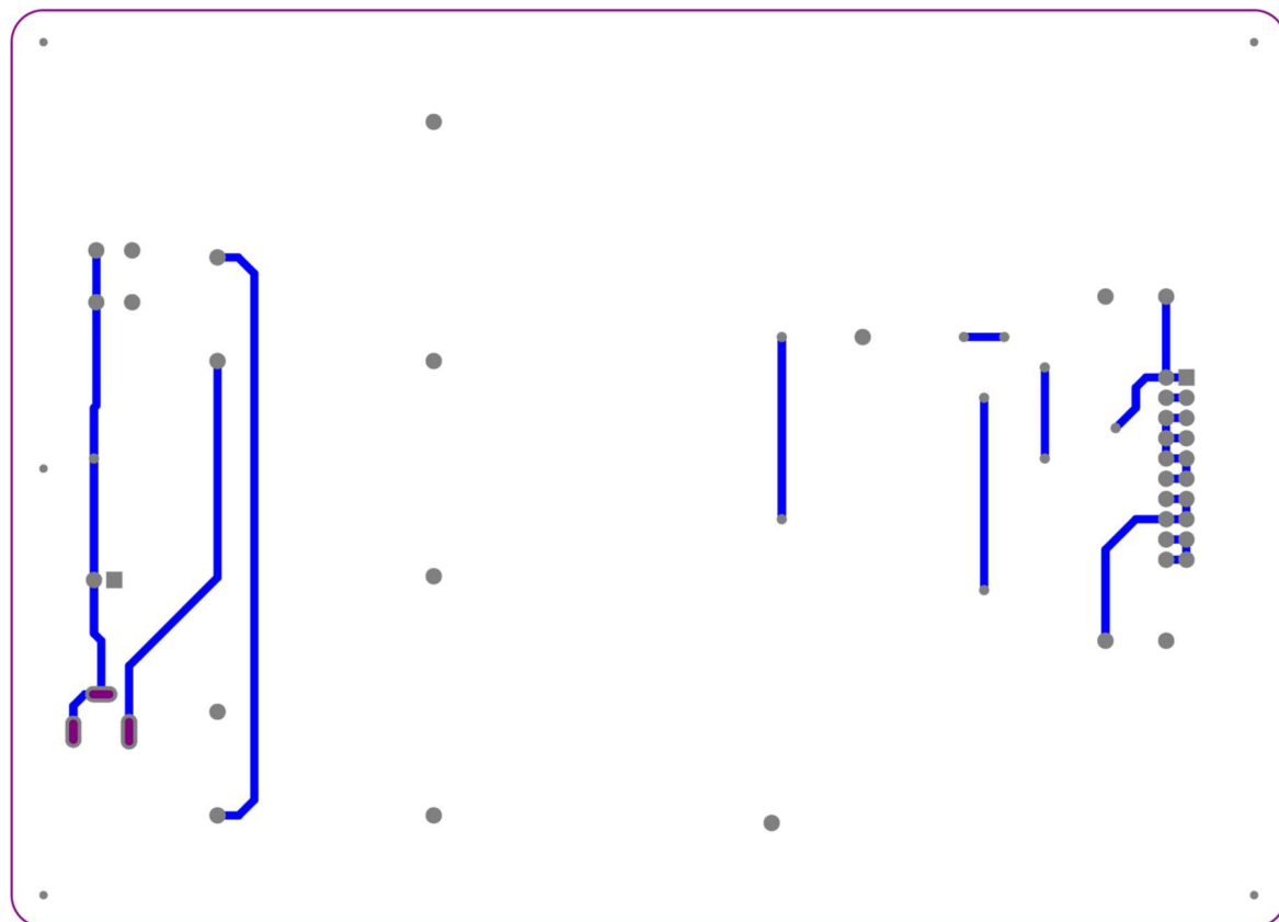
図 A3-5 「パワーボード」基板図 B 面
