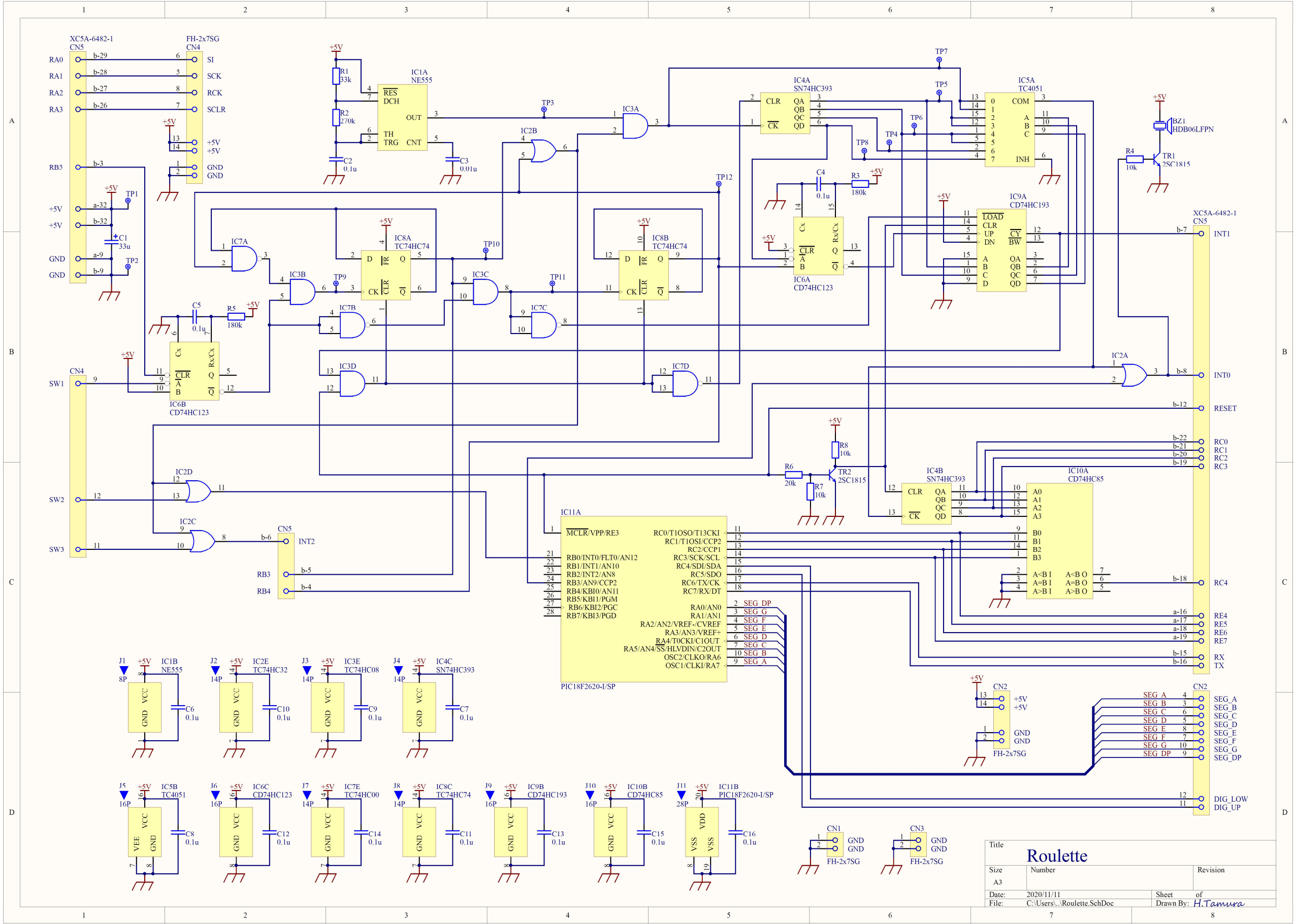
図 A2-3 「ルーレットボード」回路図
