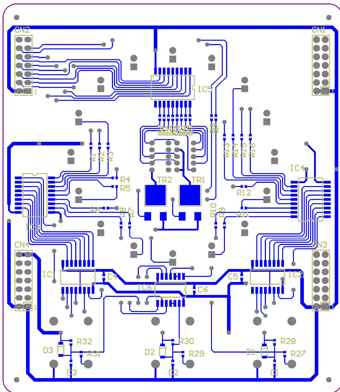
図 A2-5 「LED ディスプレイボード」 基板図 B 面
