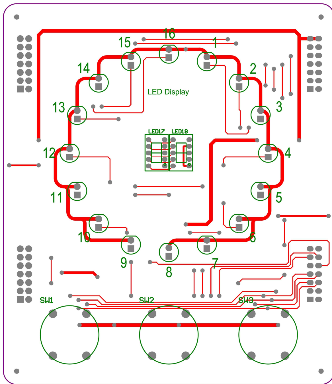
図 A2-4 「LED ディスプレイボード」基板図 A 面
