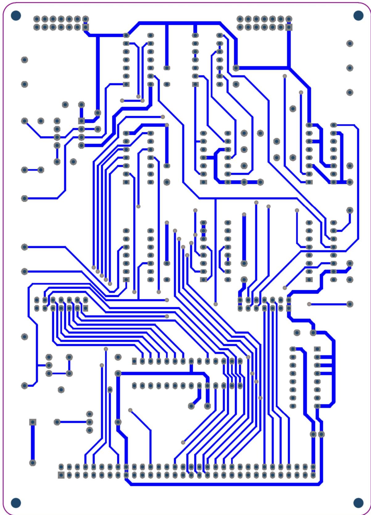
図 A2-2 「ルーレットボード」基板図 B 面
