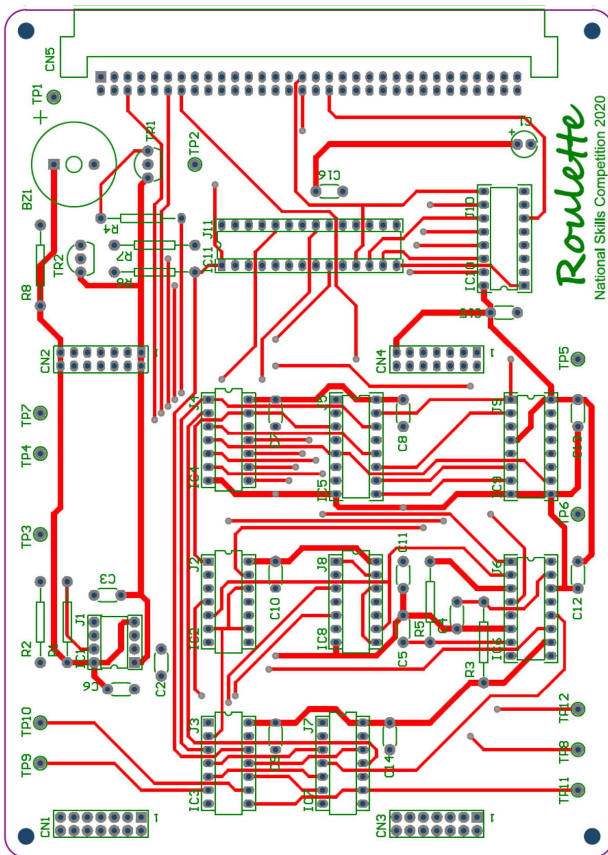
図 A2-1 「ルーレットボード」基板図 A 面
