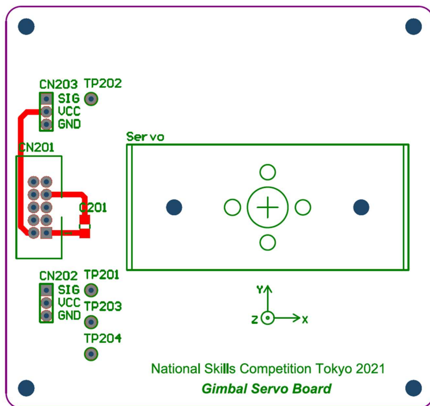
図 A2-3 「サーボボード」基板図 A 面
