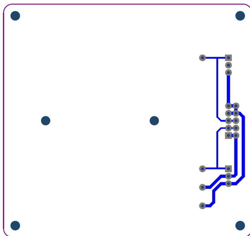
図 A2-4 「サーボボード」基板図 B 面
