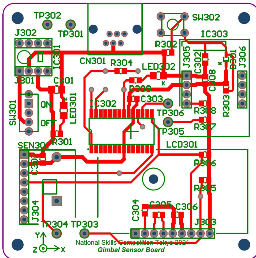
図 A2-5 「センサボード」基板図 A 面
