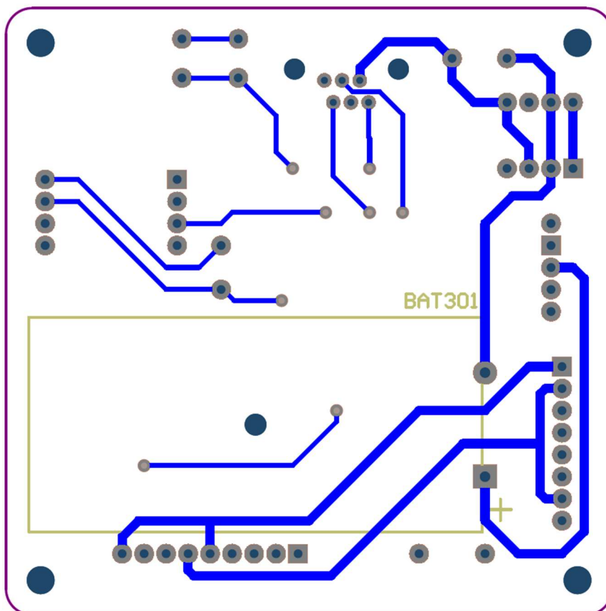
図 A2-6 「センサボード」基板図 B 面
