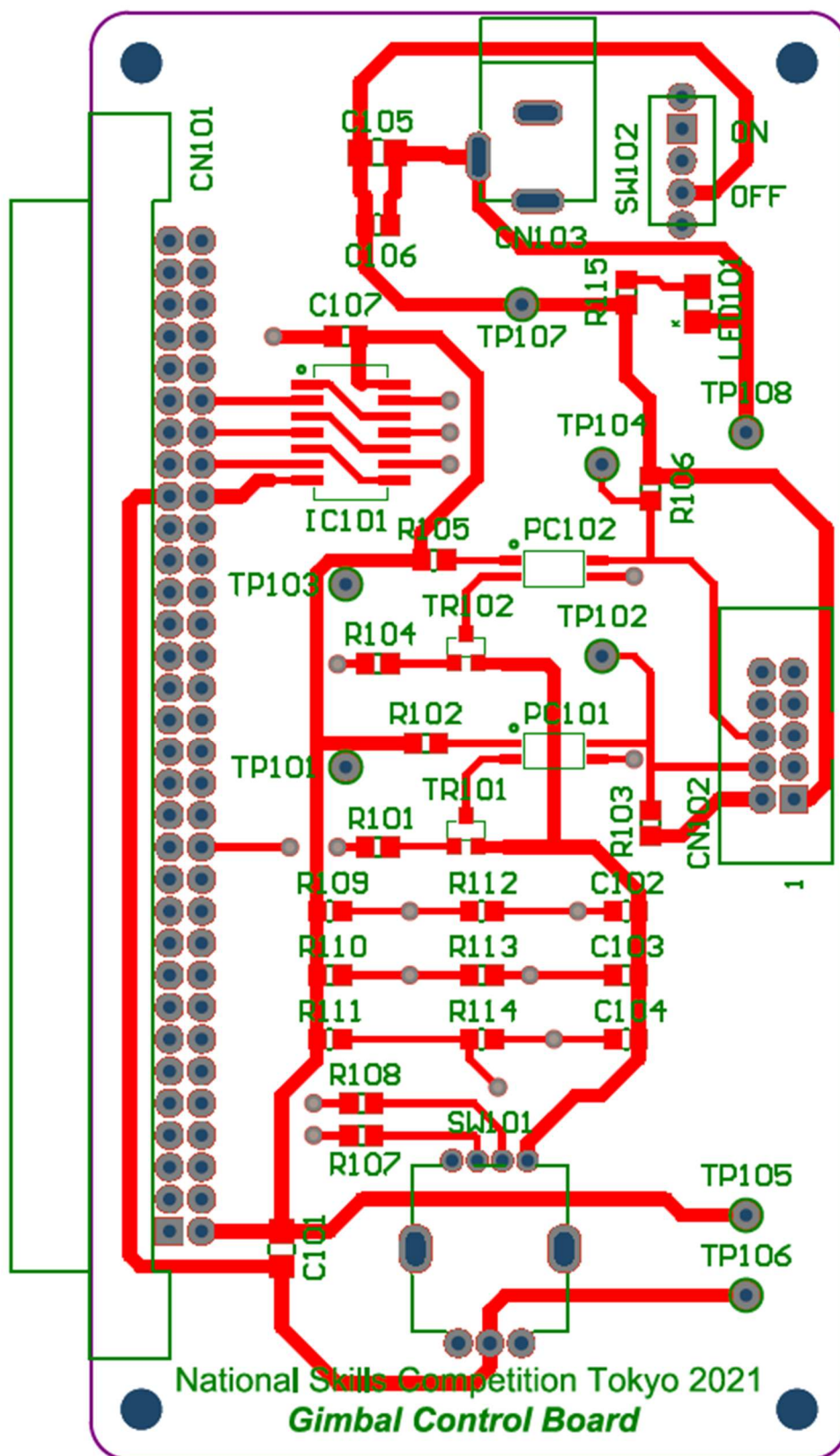
図 A2-1 「コントロールボード」 基板図 A 面
