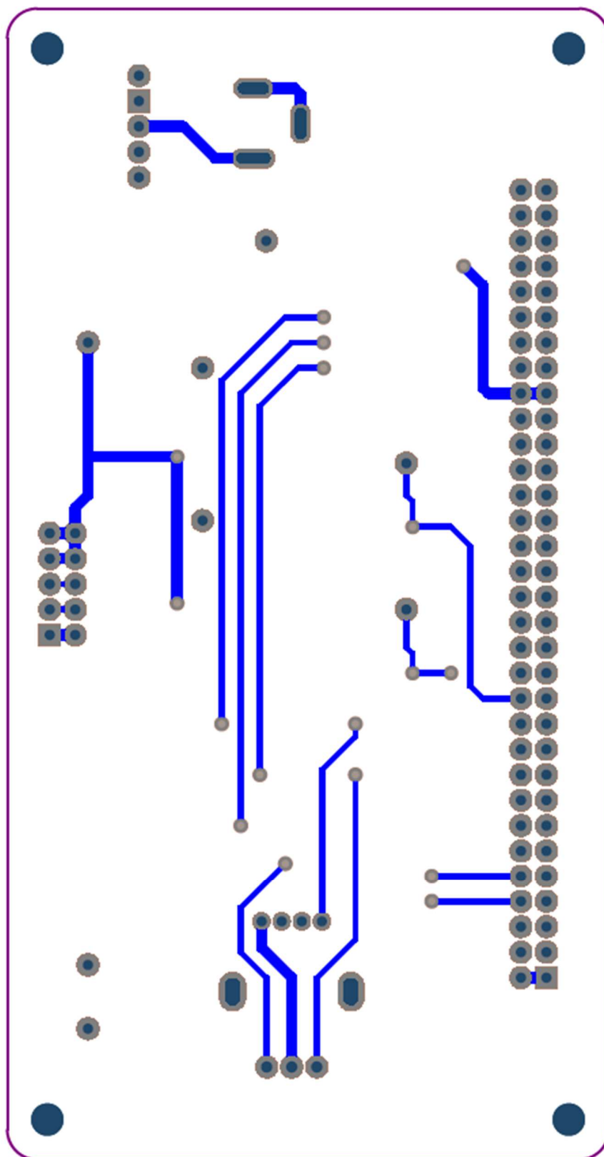
図 A2-2 「コントロールボード」基板図 B 面
