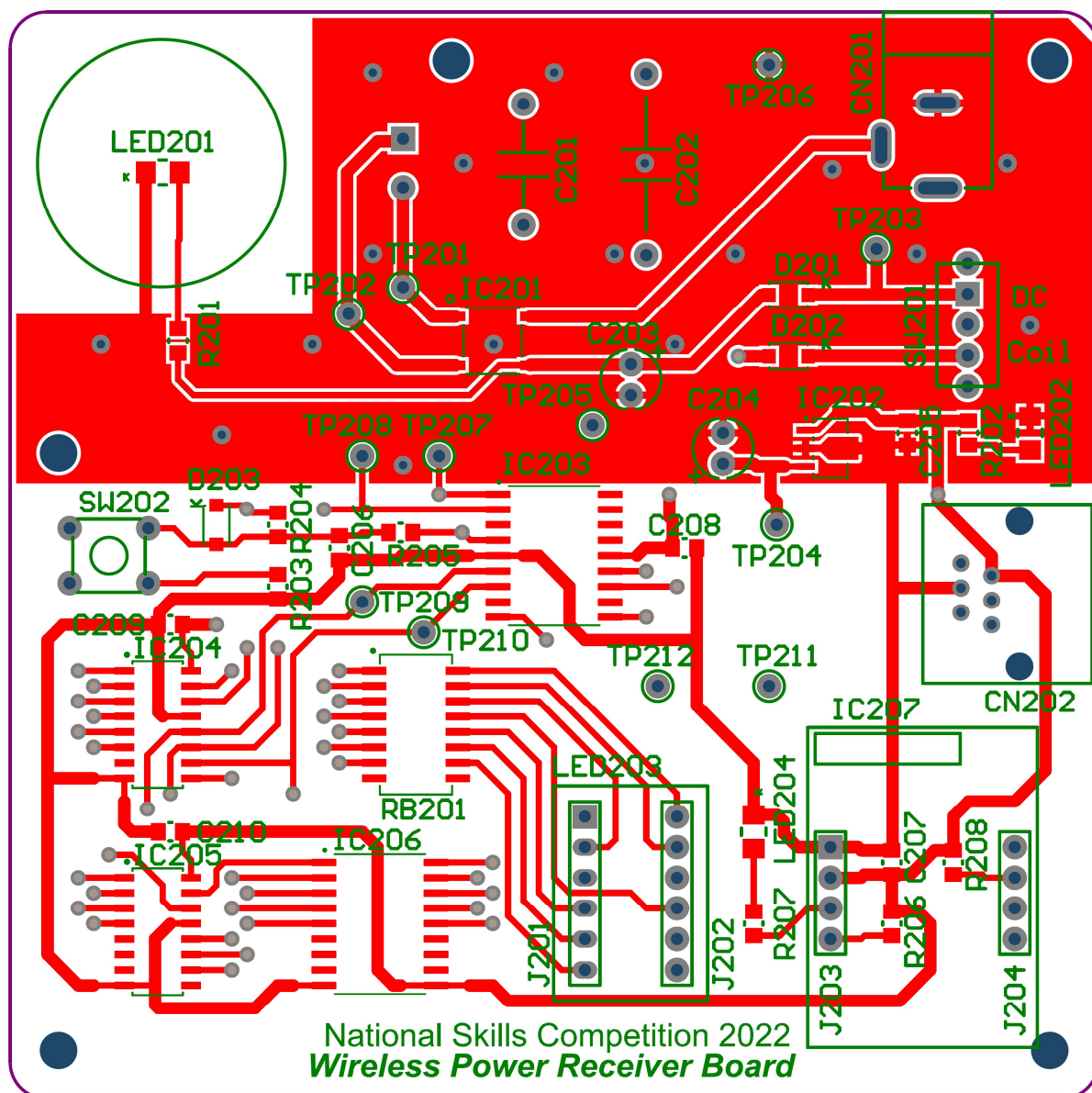
図 A2-3 「受電ボード」基板図 A 面
