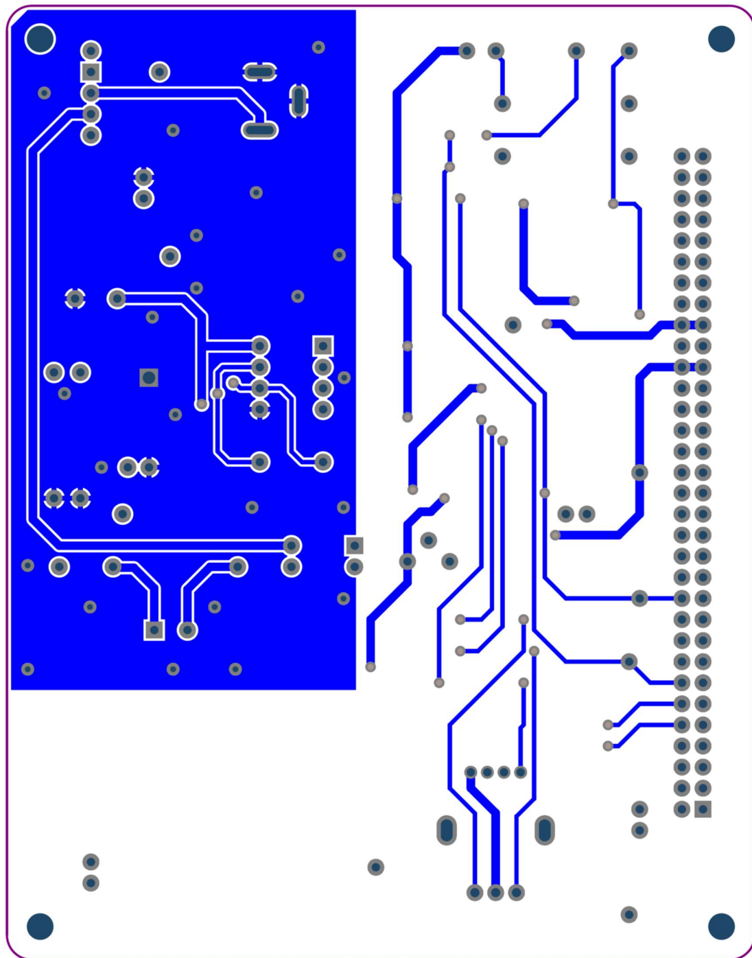
図 A2-2 「送電ボード」基板図 B 面
