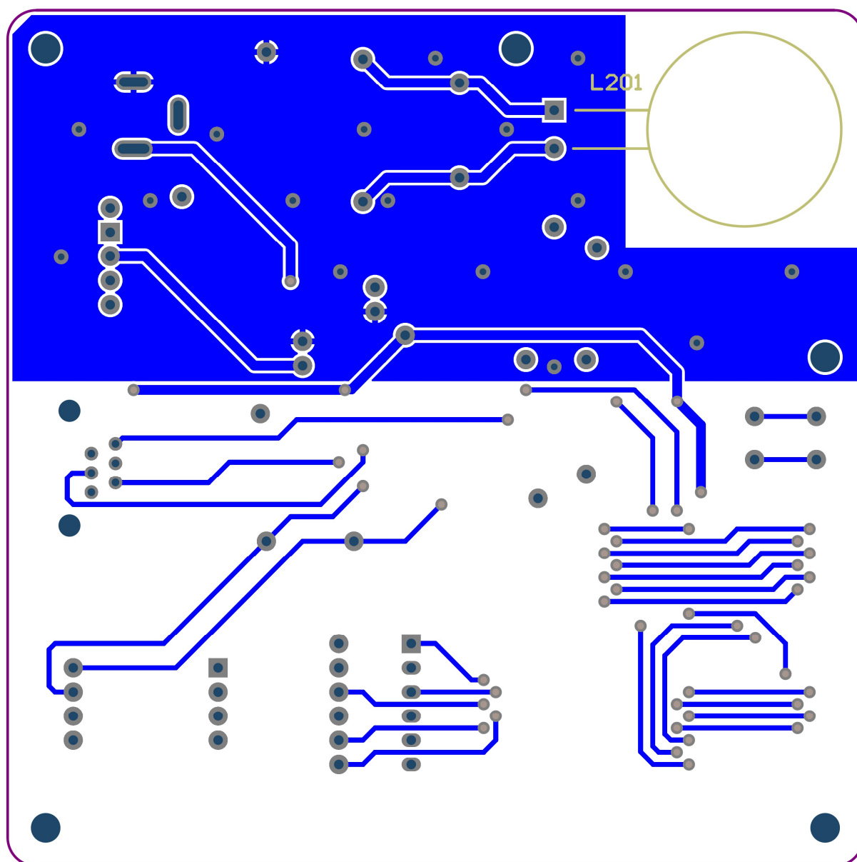
図 A2-4 「受電ボード」基板図 B 面
