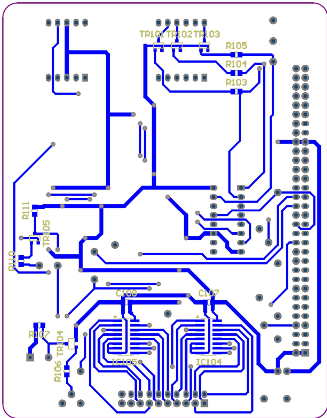
図 A2-2 「モグラ制御ボード」基板図 B 面
