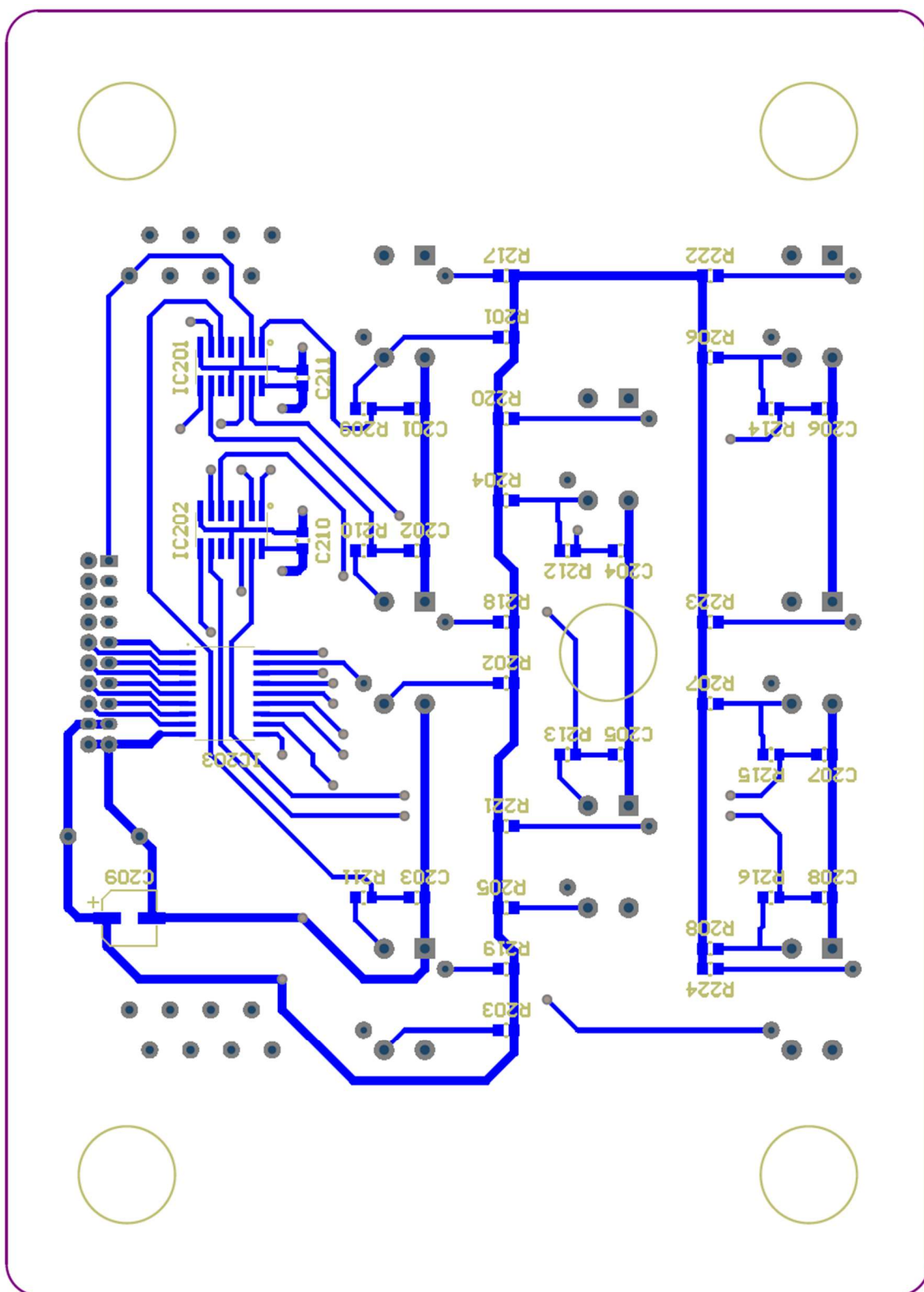
図 A2-4 「モグラたたきボード」 基板図 B 面
