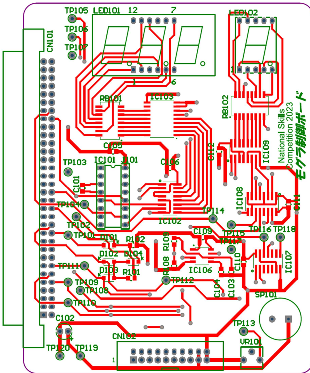
図 A2-1 「モグラ制御ボード」基板図 A 面
