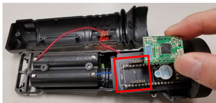
図 7.5 手順5：ZIG-100B の取付け
