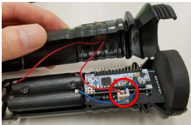
図 7.4 手順4：ケースと2P コネクタの取外し
