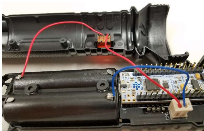
図 7.6 配線図
