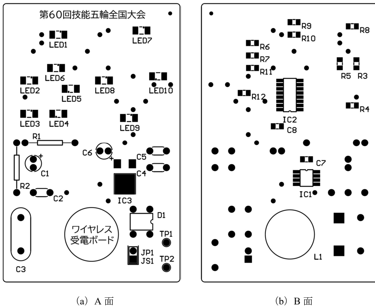
図 A2.1 ワイヤレス受電ボード部品配置図（原寸×1.4）
