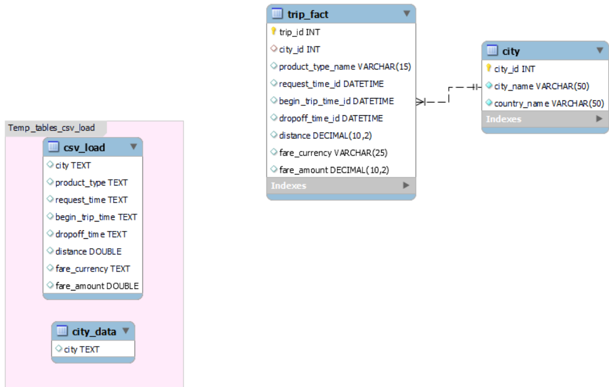
Figure 7: ER Diagram
