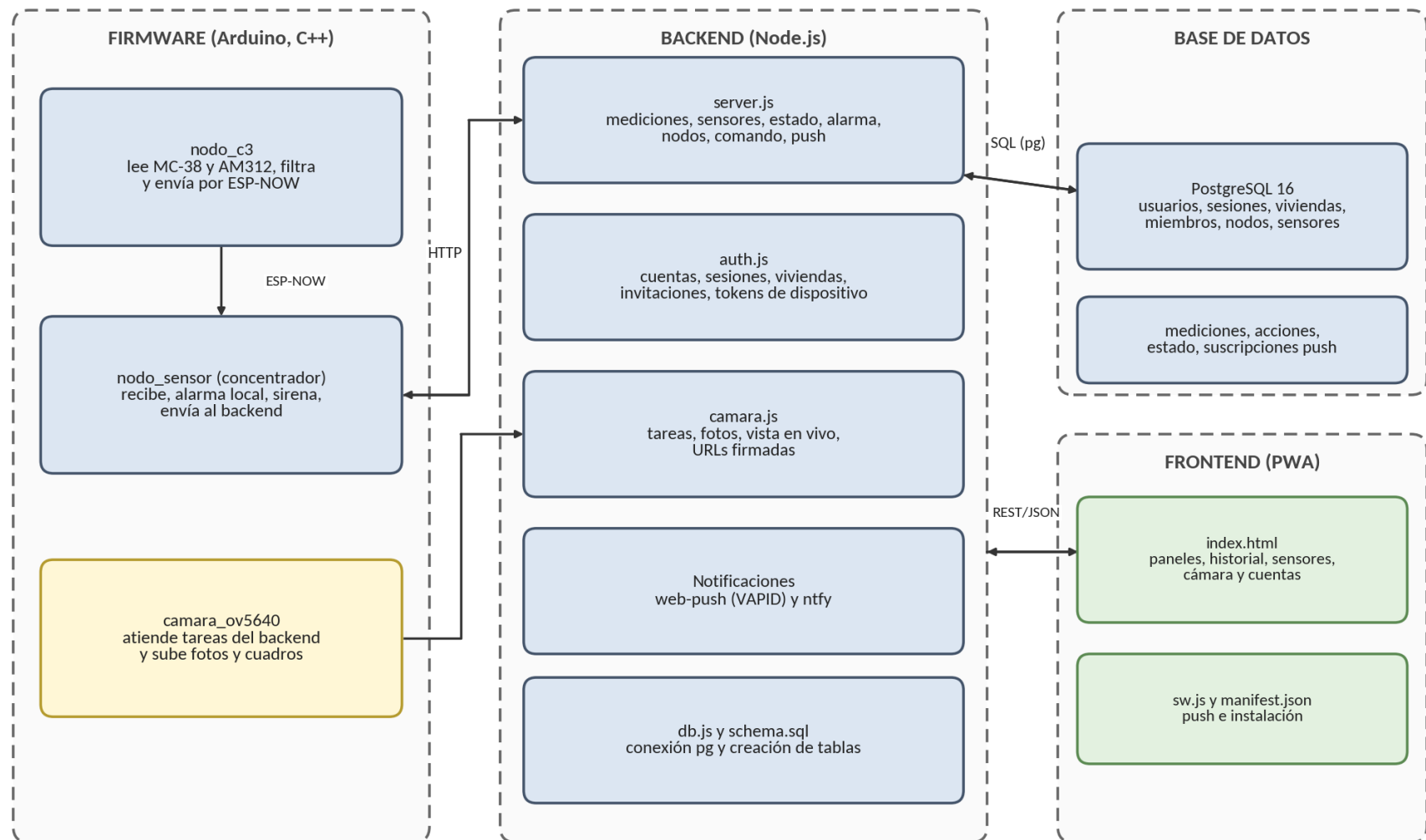
Figura 3. Diagrama de módulos de software.
