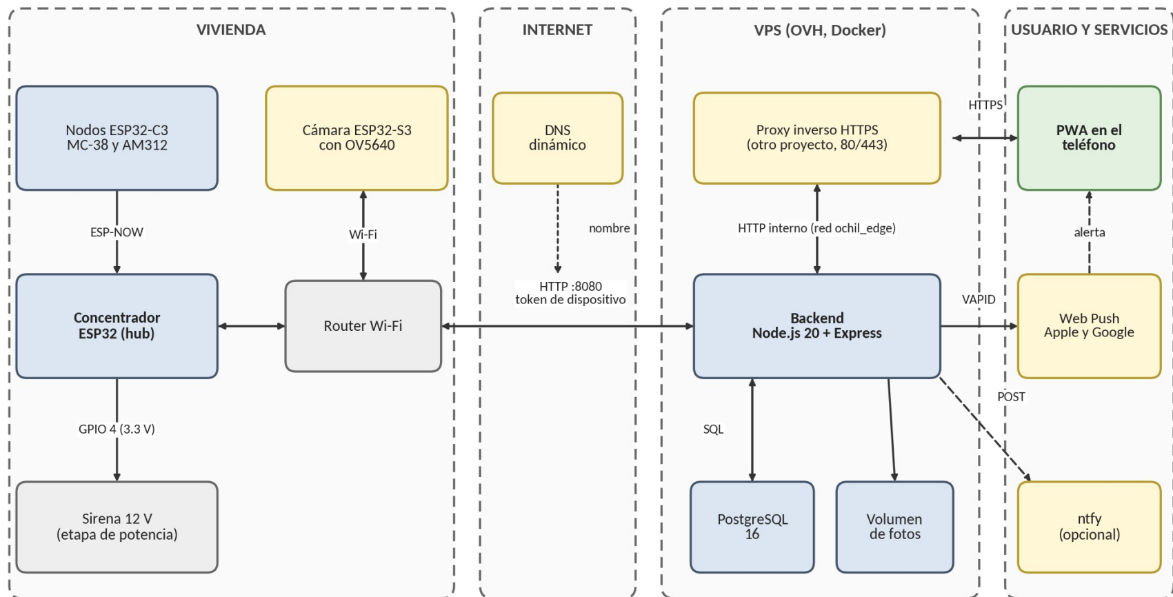
Figura 1. Arquitectura general y despliegue. En azul los componentes propios, en amarillo los servicios o equipos de terceros, en verde la aplicación del usuario y en gris el equipo pasivo.
