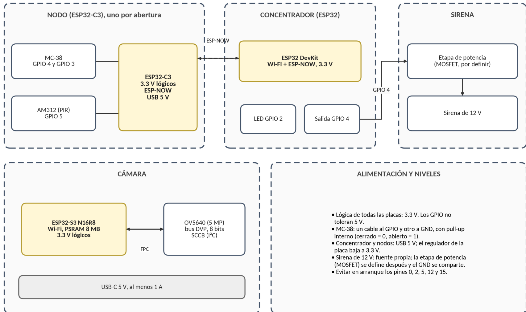
Figura 2. Diagrama de hardware con pines y niveles de voltaje.
