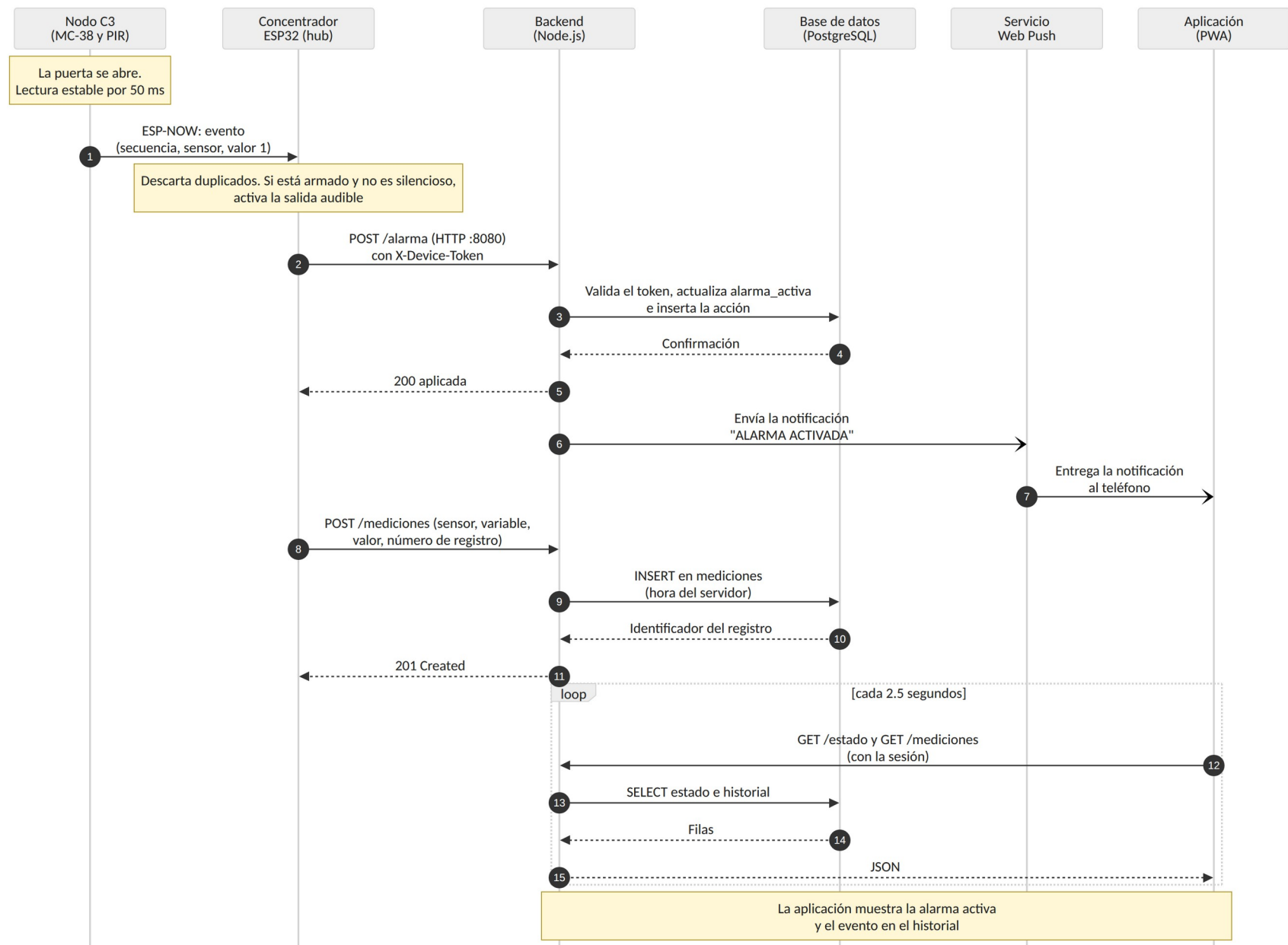
Figura 4. Flujo de una alarma: del contacto al teléfono.
