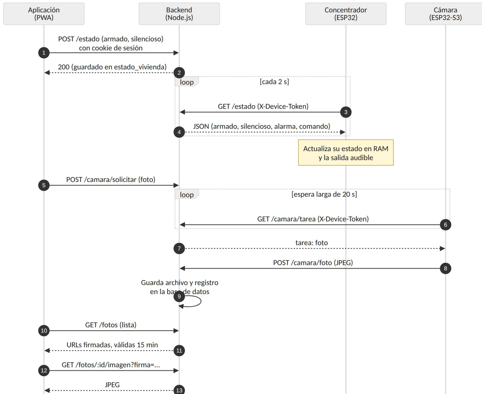
Figura 5. Flujo de control y de la cámara.
