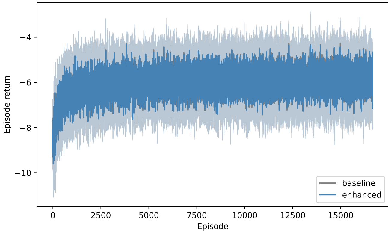
Fig. 1 - Courbes d'apprentissage (5 seeds, CI95 ombree)
