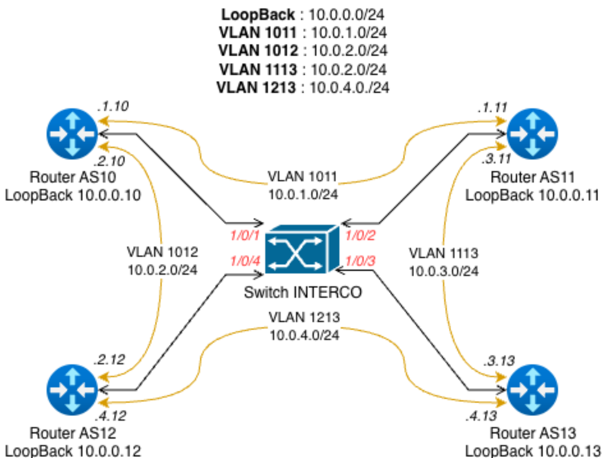
Figure 2: Schéma technique du réseau d'interconnexion
