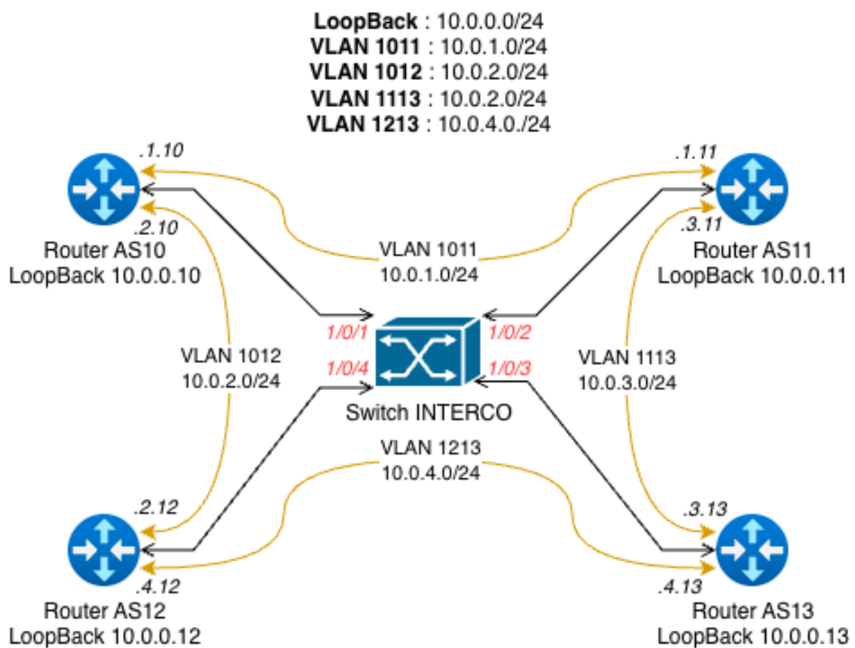
Figure 11: Schéma technique du réseau d'interconnexion
