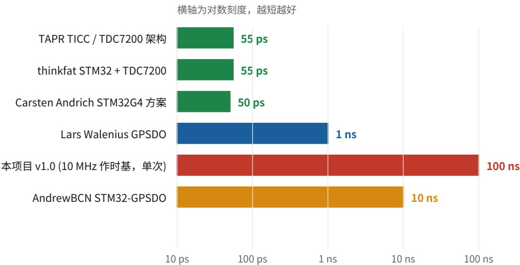
图 3 各项目的时差测量分辨率，对数横轴（注意这不等于输出 ADEV）
