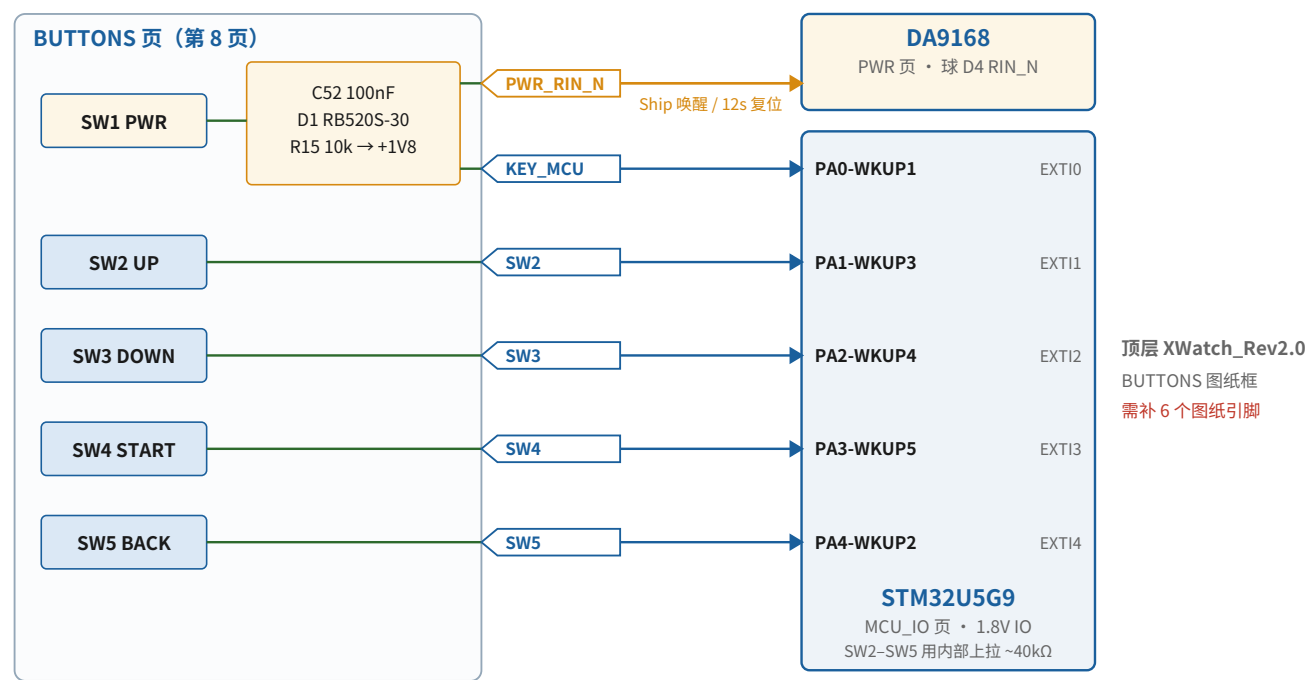
图 2 按键系统连接框图（修改后）
