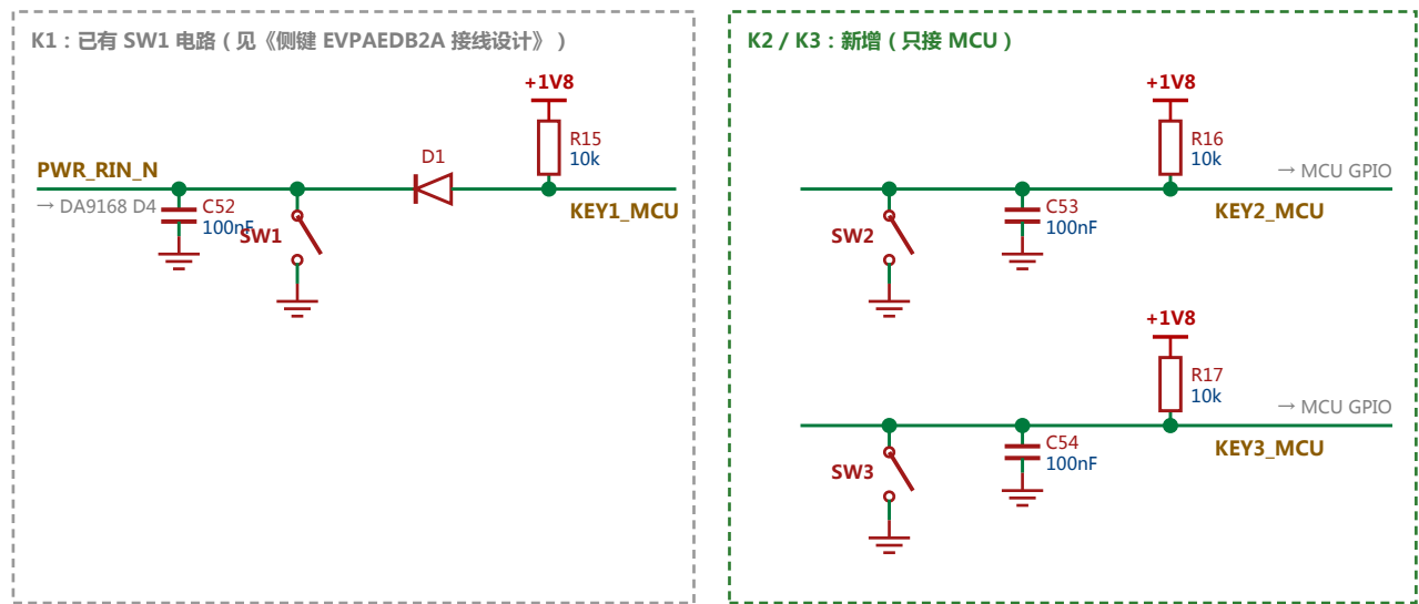
新增 2 × EVPAEDB2A + 2 × 10k + 2 × 100nF；位号接在现有编号之后，画图时按实际情况调整。 图 4 三键电路：K1 沿用已有电路，K2 / K3 只接 MCU GPIO
