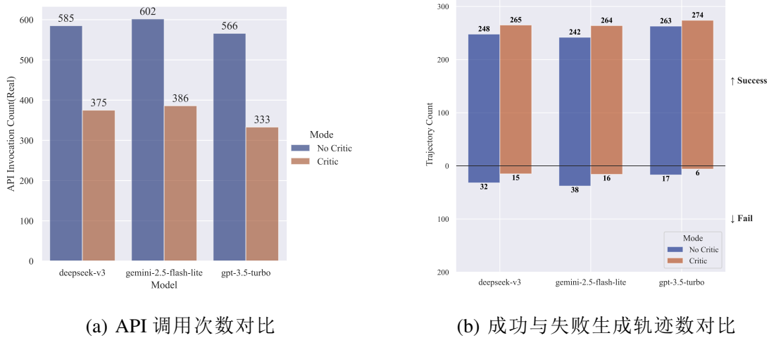
图 3-8 Critic 角色在轨迹生成阶段对 API 调用次数与成功率的影响对比
