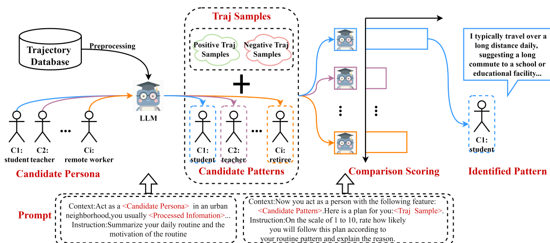
图 3-1 基于对比评分的模式评估机制
