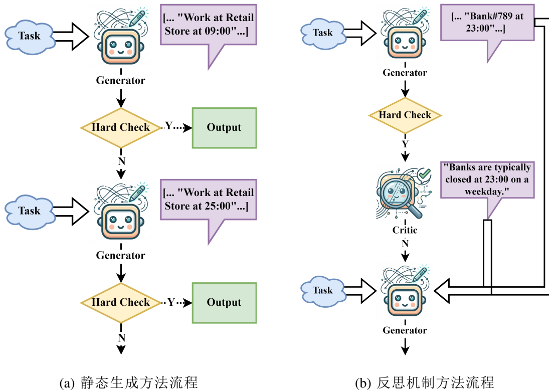
图 3-7 静态生成与反思机制轨迹生成流程对比
