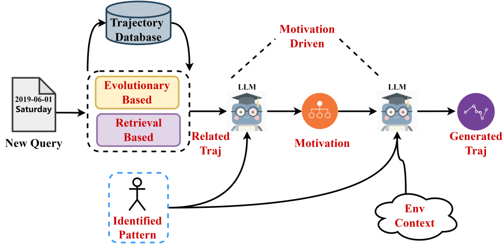
图 3-2 动机驱动的活动轨迹生成示意图
