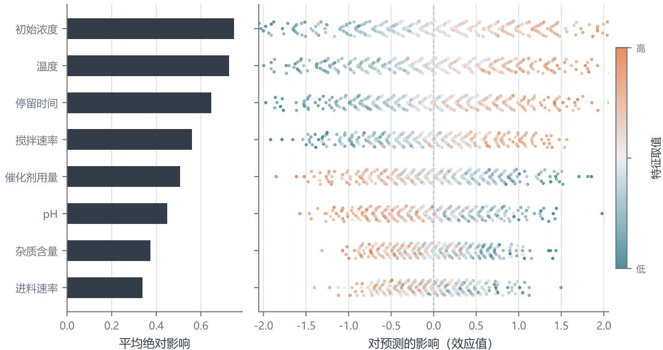
特征重要性与样本效应分布
