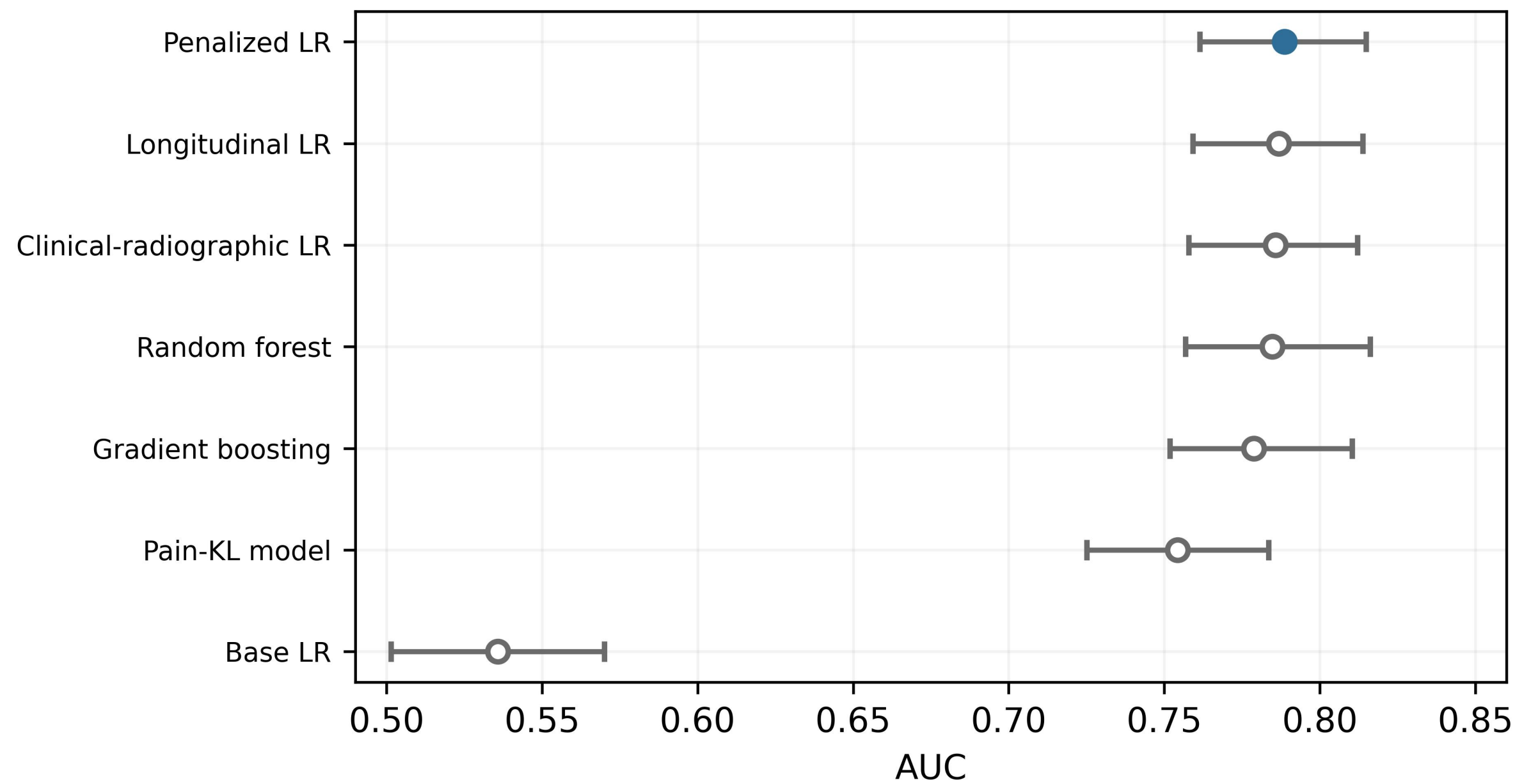
A. Candidate-model AUC
