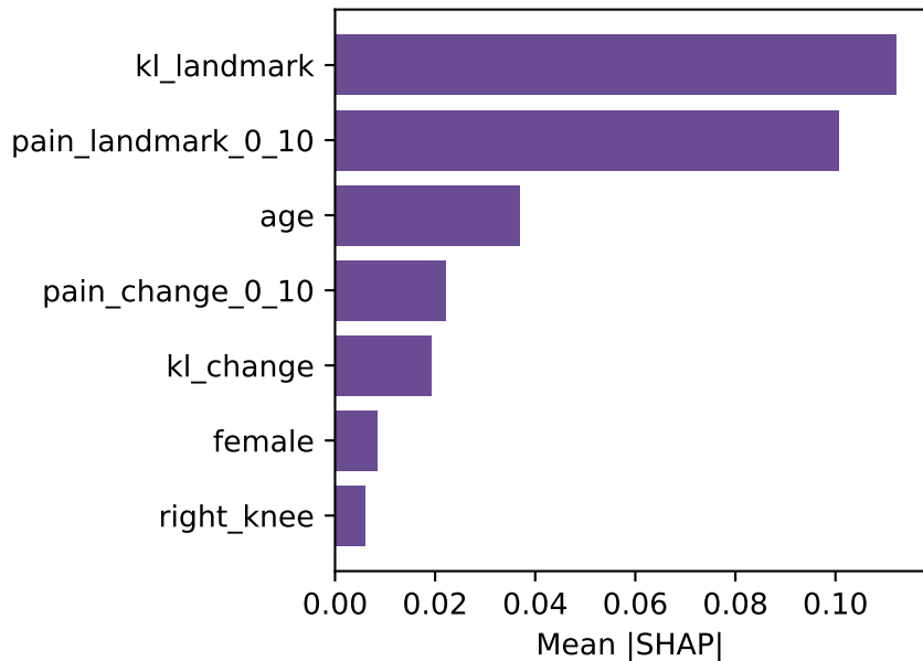
A. Global importance
