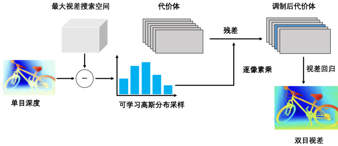
图 3-2 基于单目先验的代价体高斯调制器设计图
