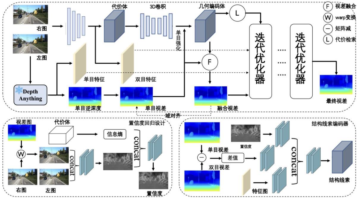
图 3-1 PGStereo 的总体架构
