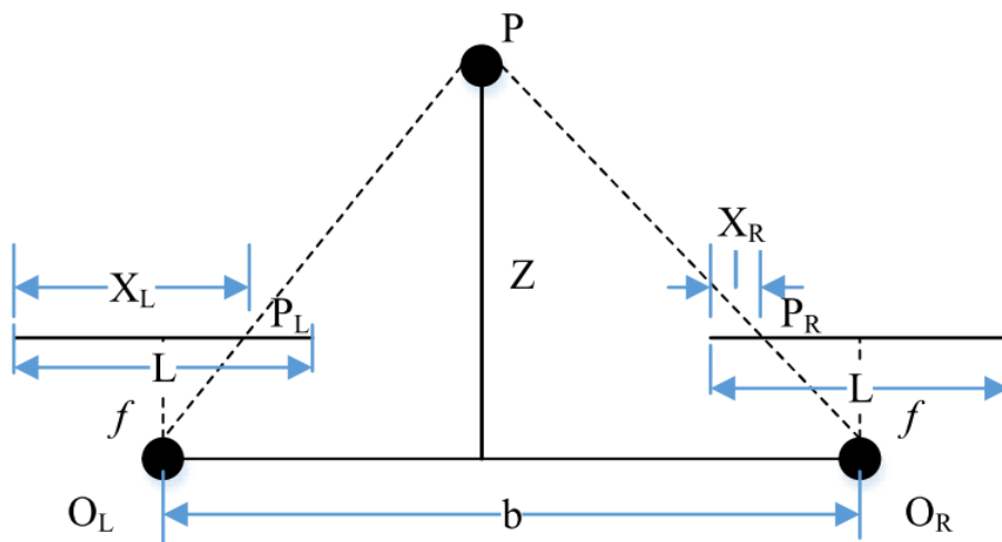
图 2-1 立体匹配相机成像模型
