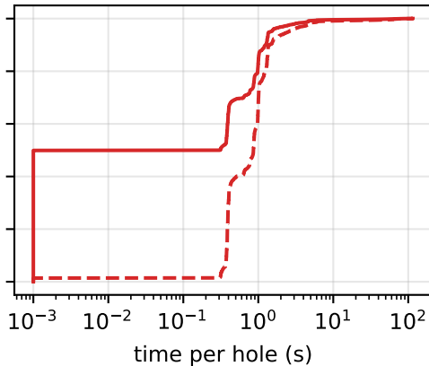
QF_LIA
