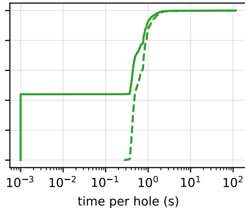
QF_LRA
