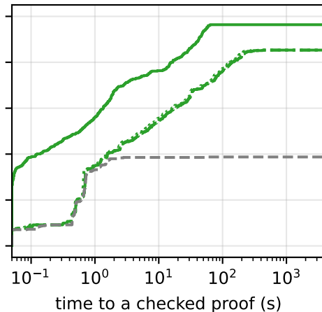
QF_LRA (524)
