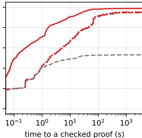
QF_LIA (2541)
