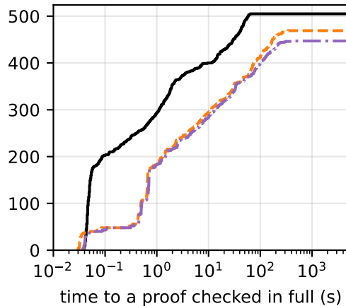
QF_LRA (524 benchmarks)
