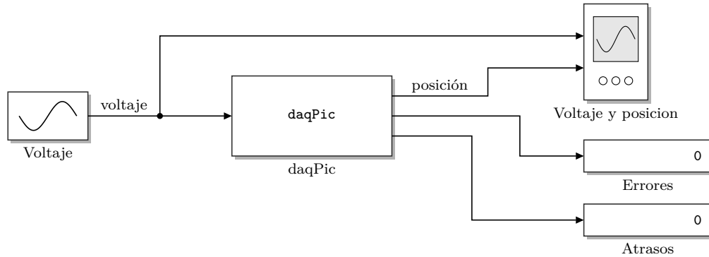
Figura 3: Modelo DaqPicPrueba ( crear_modelo.m ) con la versión en un bloque. Parámetros de daqPic : 0.001, 1. Salidas, de arriba abajo: posición [cuentas], errores de comunicación y pasos atrasados.
