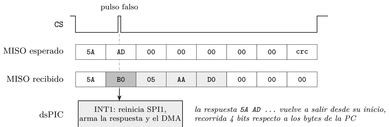
Figura 6: Respuesta dañada por un pulso falso en CS (resultados/2026-10-06_dock/visor_dspic_1khz). Se esperaba 5A AD 00 00 00 00 00 00 y se recibió 5A B0 05 AA D0 00 00 00: a partir del byte 1 reaparecen 5A AD desplazados medio byte.
