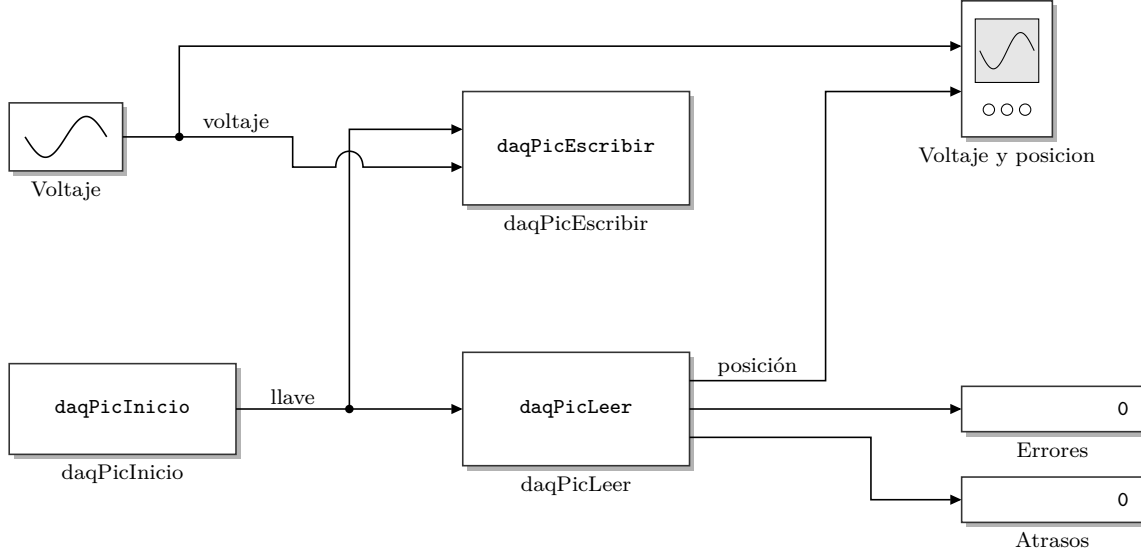
Figura 4: Modelo DaqPicBloquesPrueba ( crear_modelo_bloques.m ) con la versión en tres bloques. Parámetros de daqPicInicio : 0.001, 1; daqPicEscribir y daqPicLeer no tienen parámetros y heredan el periodo de muestreo. Entradas de daqPicEscribir : llave y voltaje; salidas de daqPicLeer : las mismas de daqPic .
