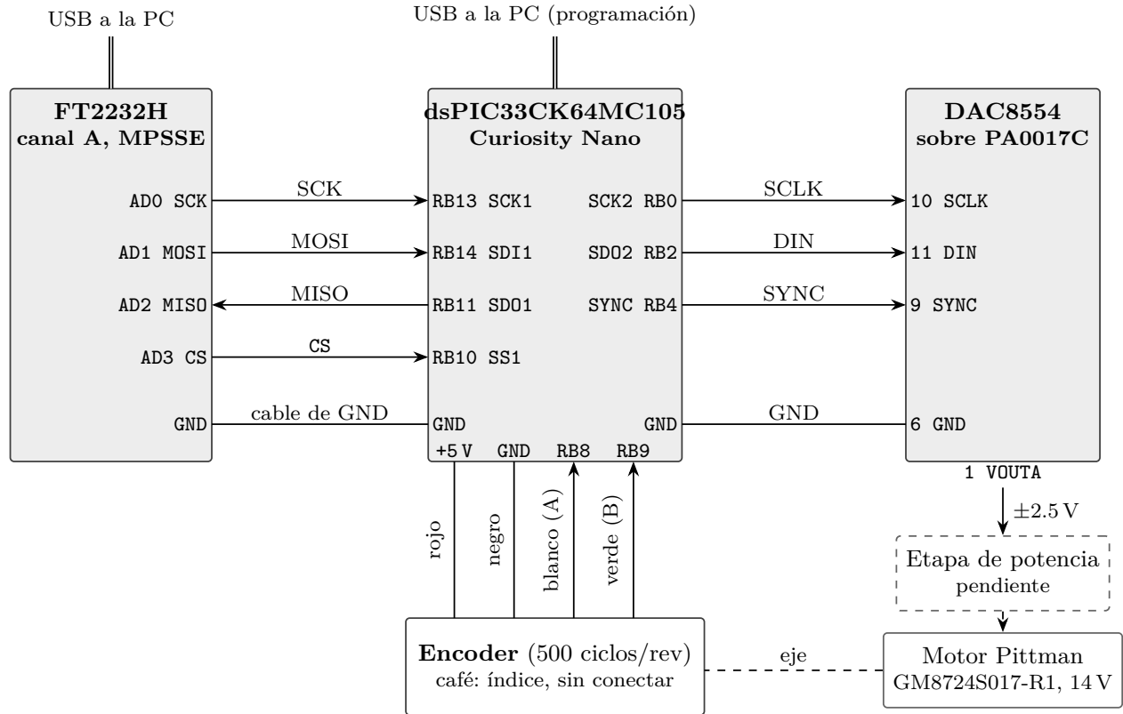
Figura 1: Diagrama de conexiones. Las flechas indican el sentido de cada señal. Los colores del encoder deben confirmarse (ver el texto); si A y B quedan invertidos sólo cambia el signo del conteo.
