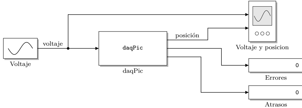
Figura 2: Modelo DaqPicPrueba ( crear_modelo.m ) con la versión en un bloque. Parámetros de daqPic : 0.001, 1. Salidas, de arriba abajo: posición [cuentas], errores de comunicación y pasos atrasados.
