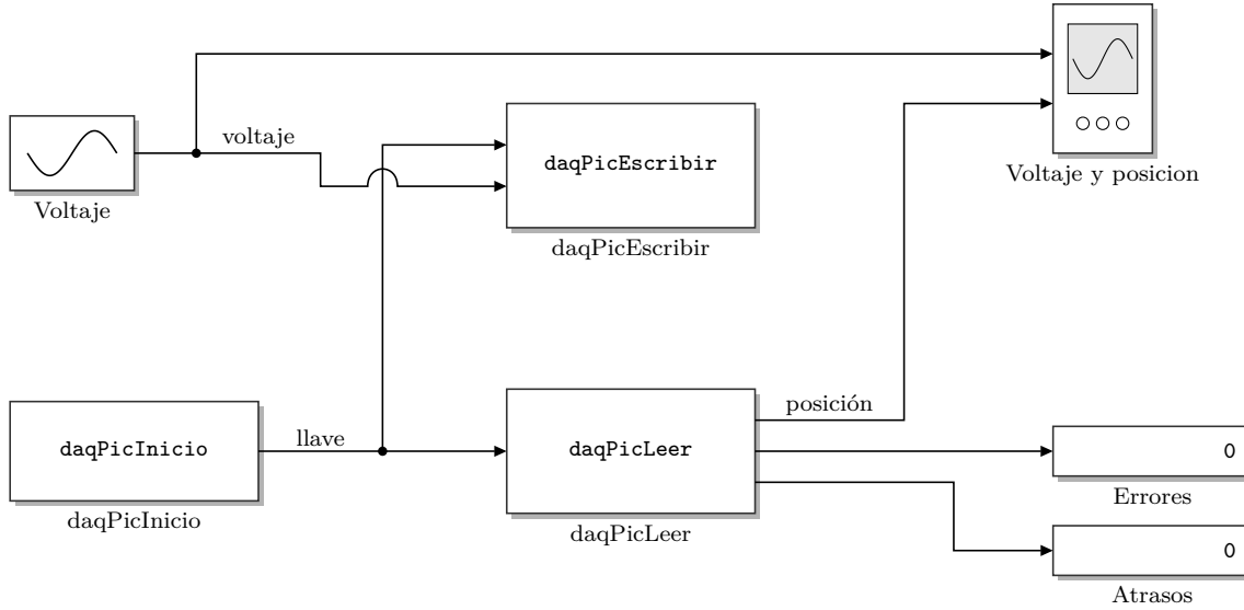
Figura 3: Modelo DaqPicBloquesPrueba ( crear_modelo_bloques.m ) con la versión en tres bloques. Parámetros de daqPicInicio : 0.001, 1; daqPicEscribir y daqPicLeer no tienen parámetros y heredan el periodo de muestreo. Entradas de daqPicEscribir : llave y voltaje; salidas de daqPicLeer : las mismas de daqPic .
