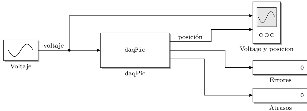
Figura 1: Modelo DaqPicPrueba ( crear_modelo.m ) con la versión en un bloque. Parámetros de daqPic : 0.001, 1. Salidas, de arriba abajo: posición [cuentas], errores de comunicación y pasos atrasados.
