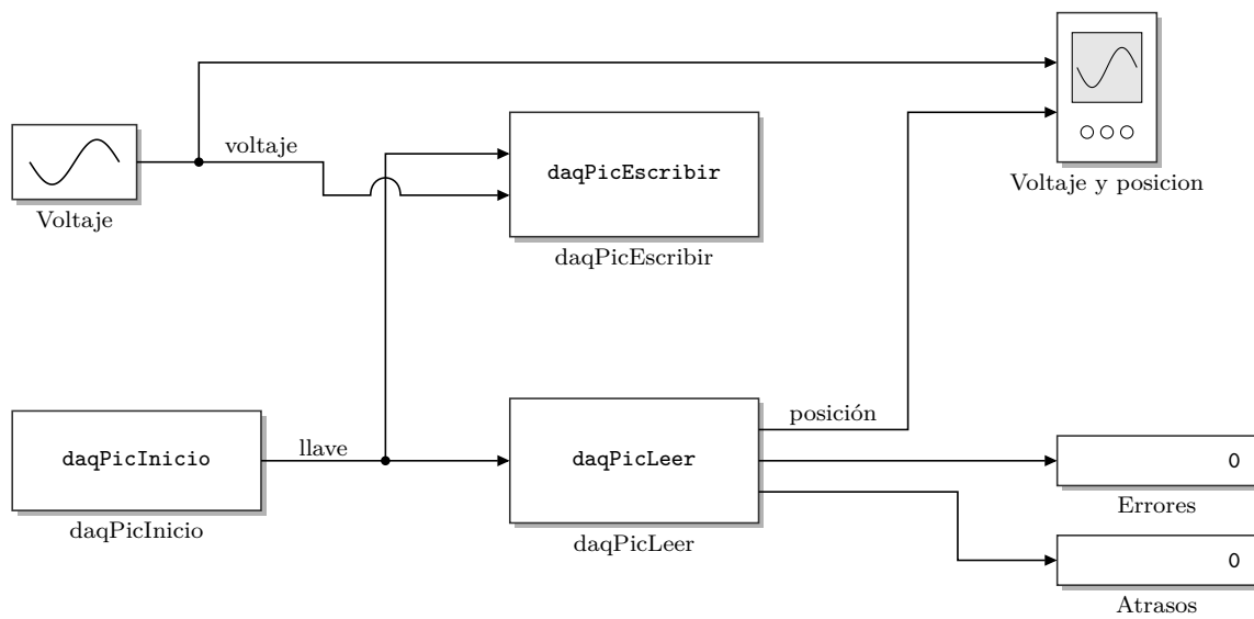
Figura 2: Modelo DaqPicBloquesPrueba ( crear_modelo_bloques.m ) con la versión en tres bloques. Parámetros de daqPicInicio : 0.001, 1; daqPicEscribir y daqPicLeer no tienen parámetros y heredan el periodo de muestreo. Entradas de daqPicEscribir : llave y voltaje ; salidas de daqPicLeer : las mismas de daqPic .
