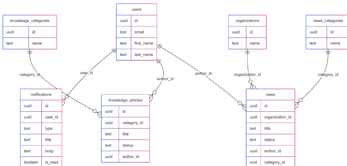
Рисунок 12 - ER-диаграмма подсистемы контента и уведомлений
