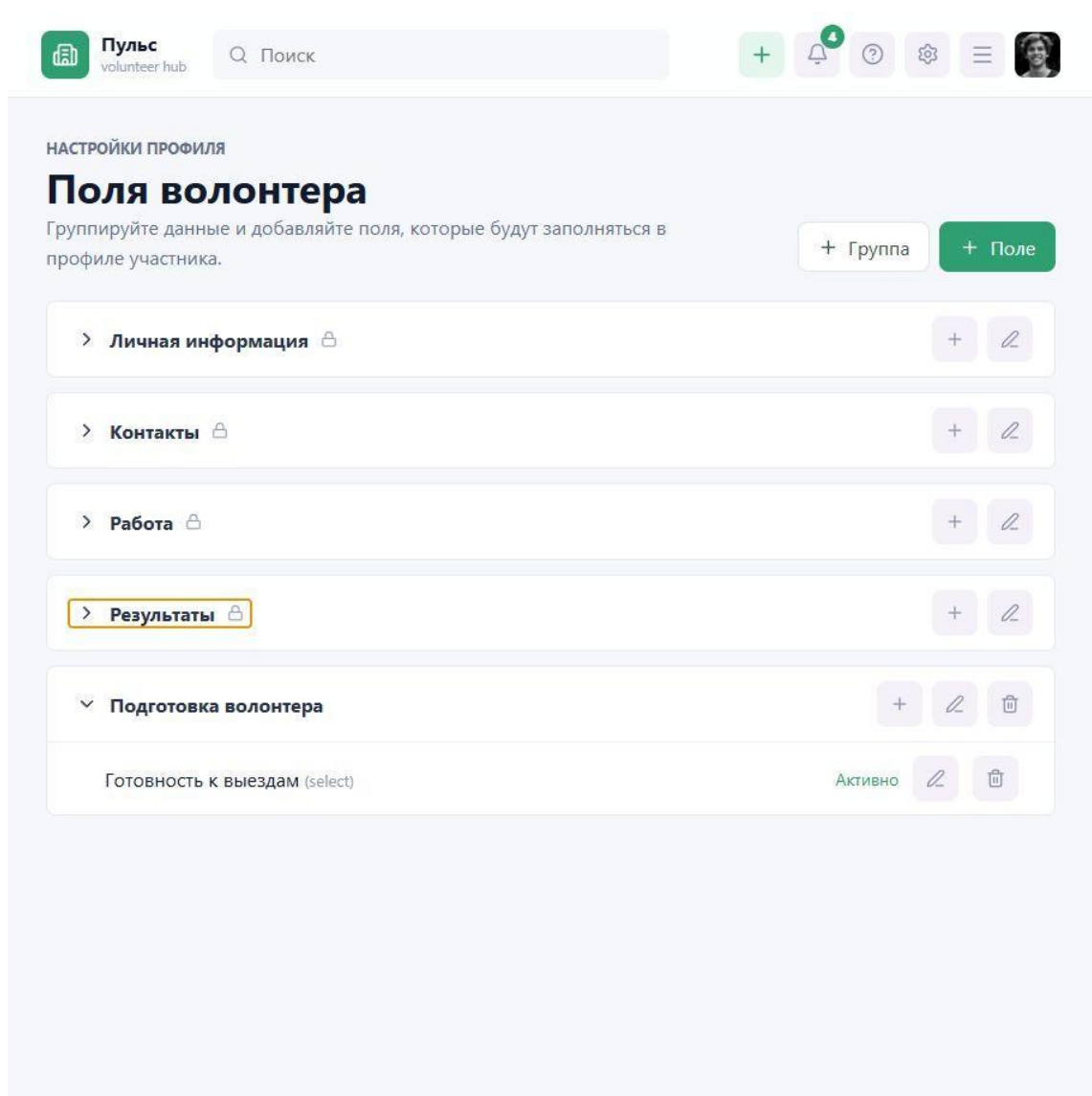
Рисунок 22 - Конструктор групп и полей профиля в системе Пульс
