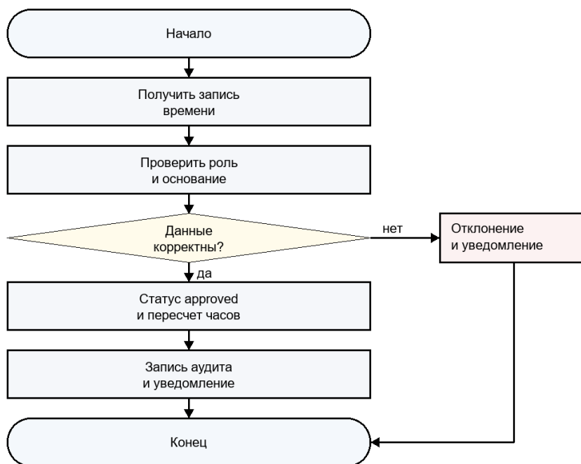
Рисунок В.2 - Подтверждение волонтерских часов
