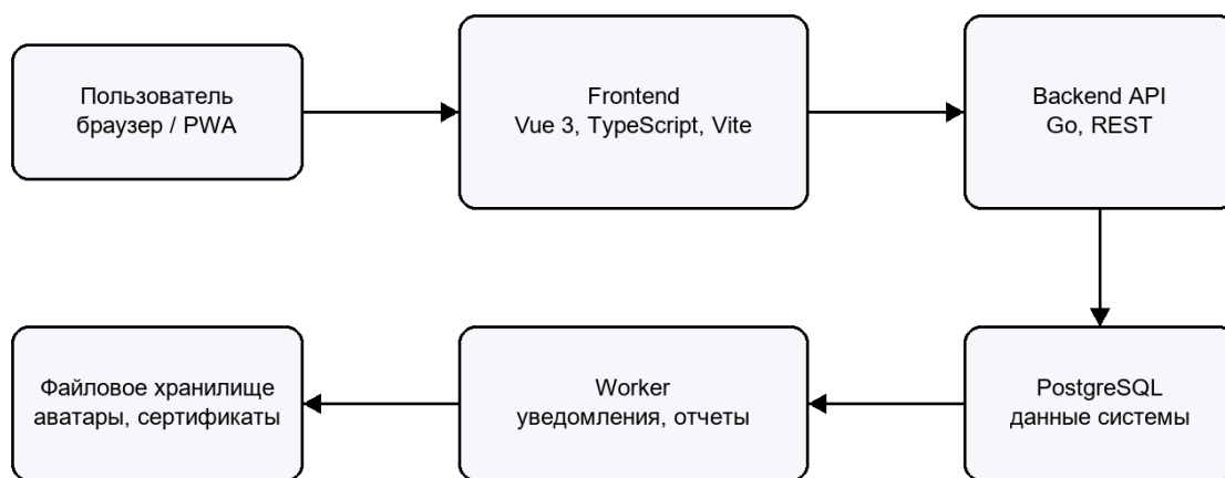
Рисунок 7 - Архитектура информационной системы Пульс
