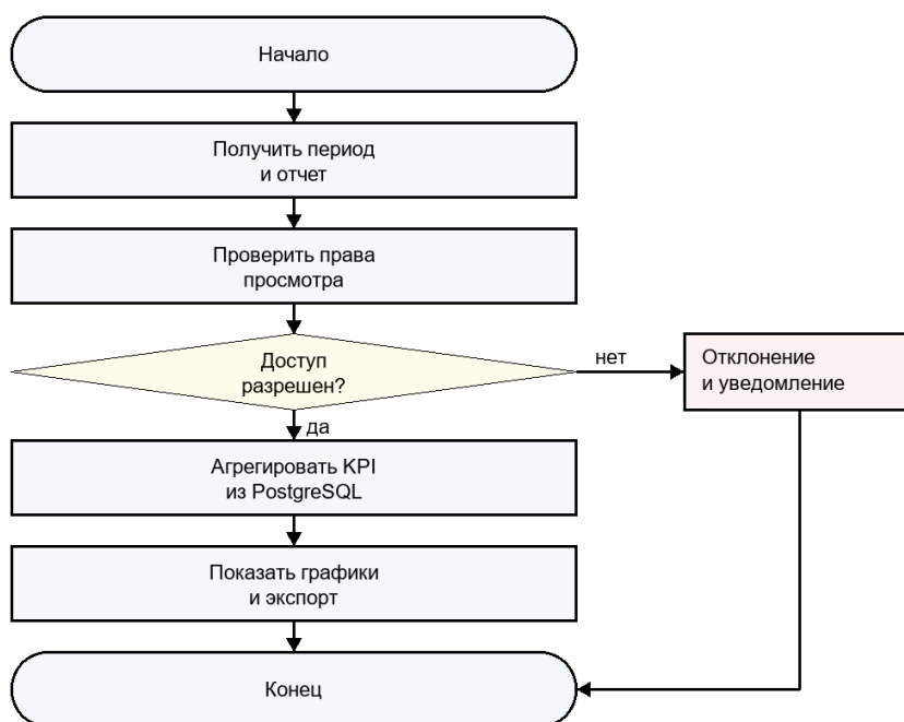
Рисунок В.5 - Формирование аналитики
