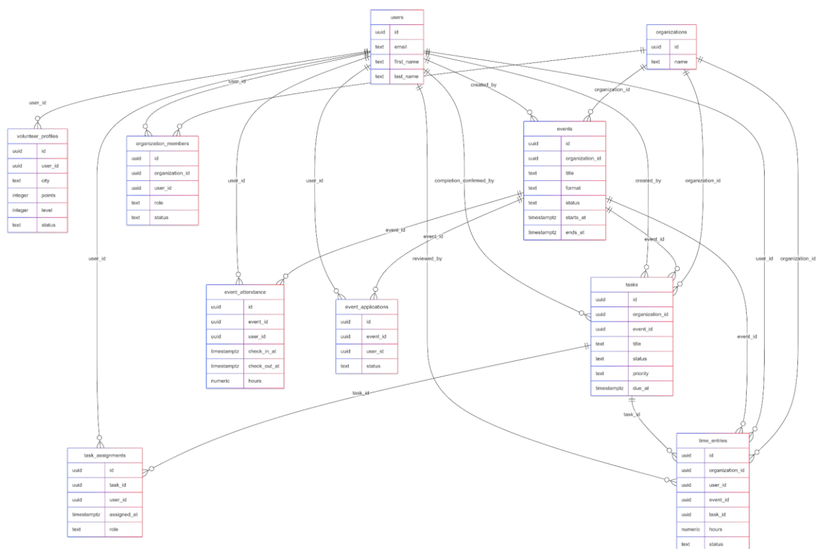
Рисунок 10 - ER-диаграмма ядра информационной системы Пульс
