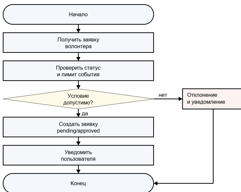
Рисунок 14 - Блок-схема алгоритма обработки заявки на мероприятие
