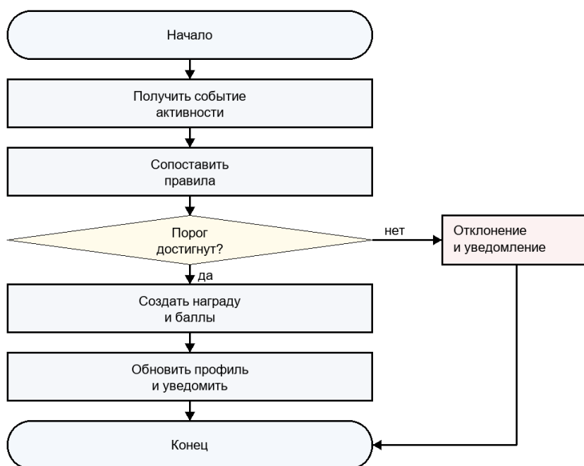
Рисунок В.3 - Начисление достижения
