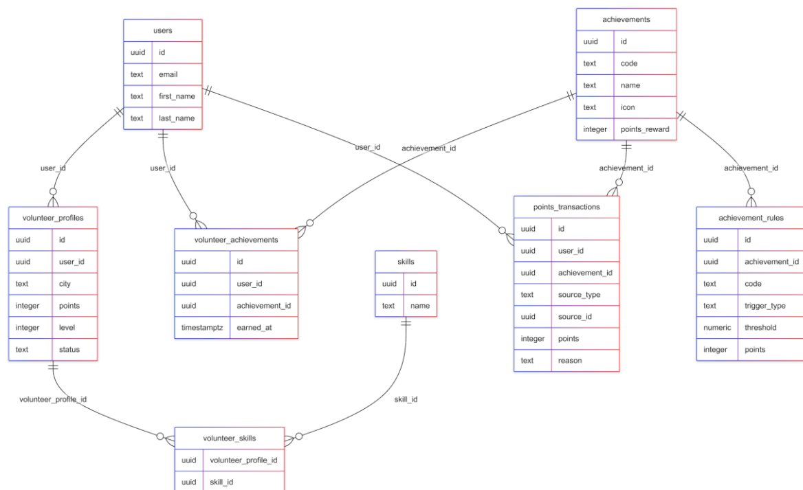
Рисунок 11 - ER-диаграмма подсистемы геймификации
