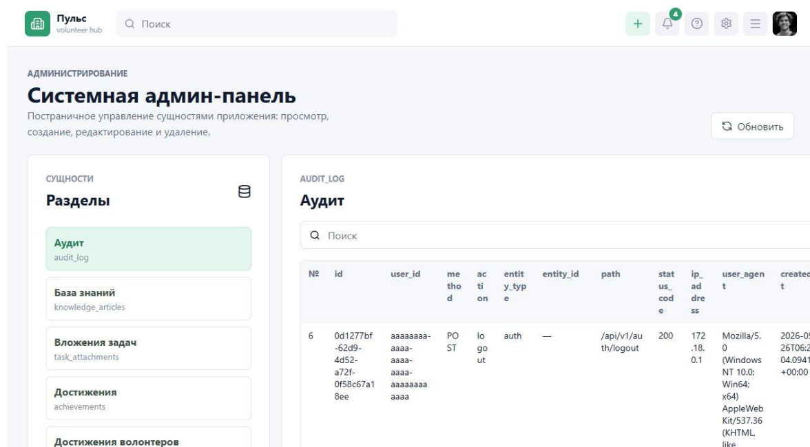
Рисунок 31 - Экран системного администрирования
