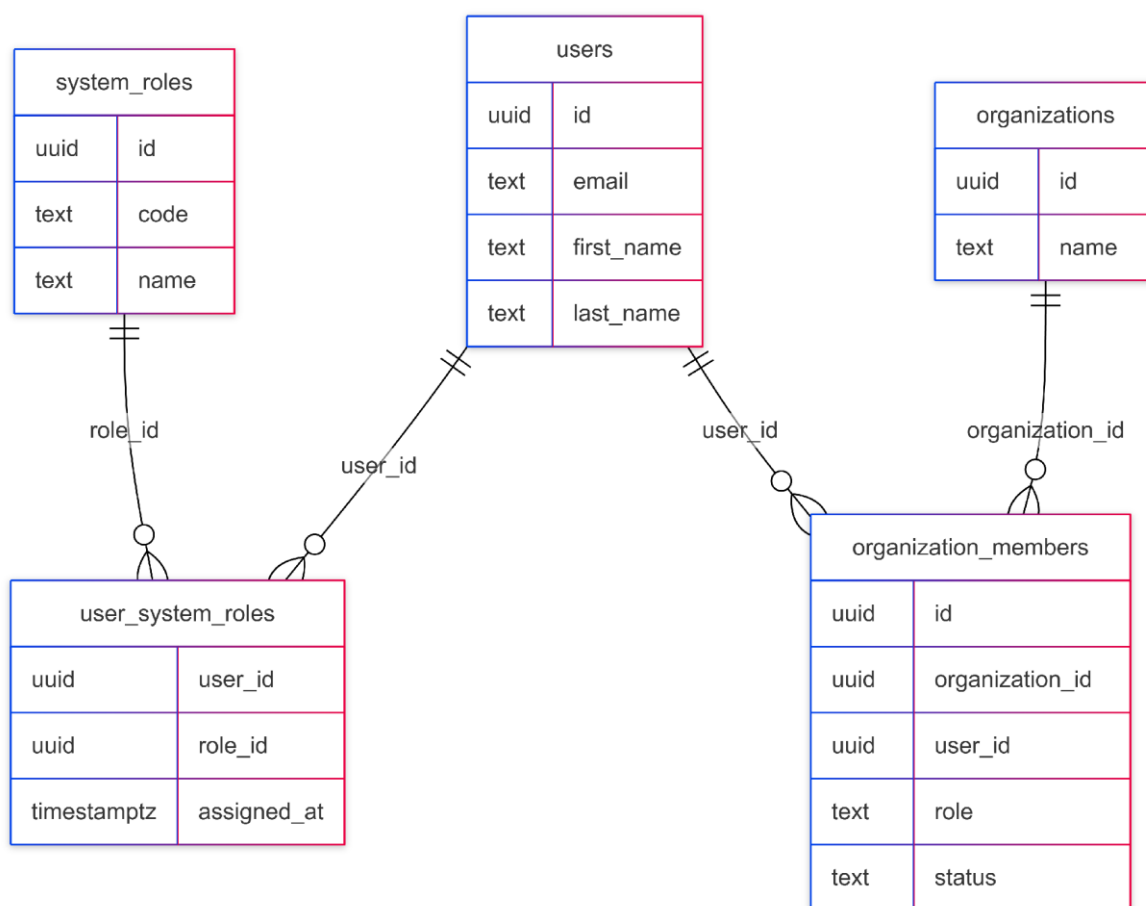
Рисунок 13 - ER-диаграмма ролей и членства
