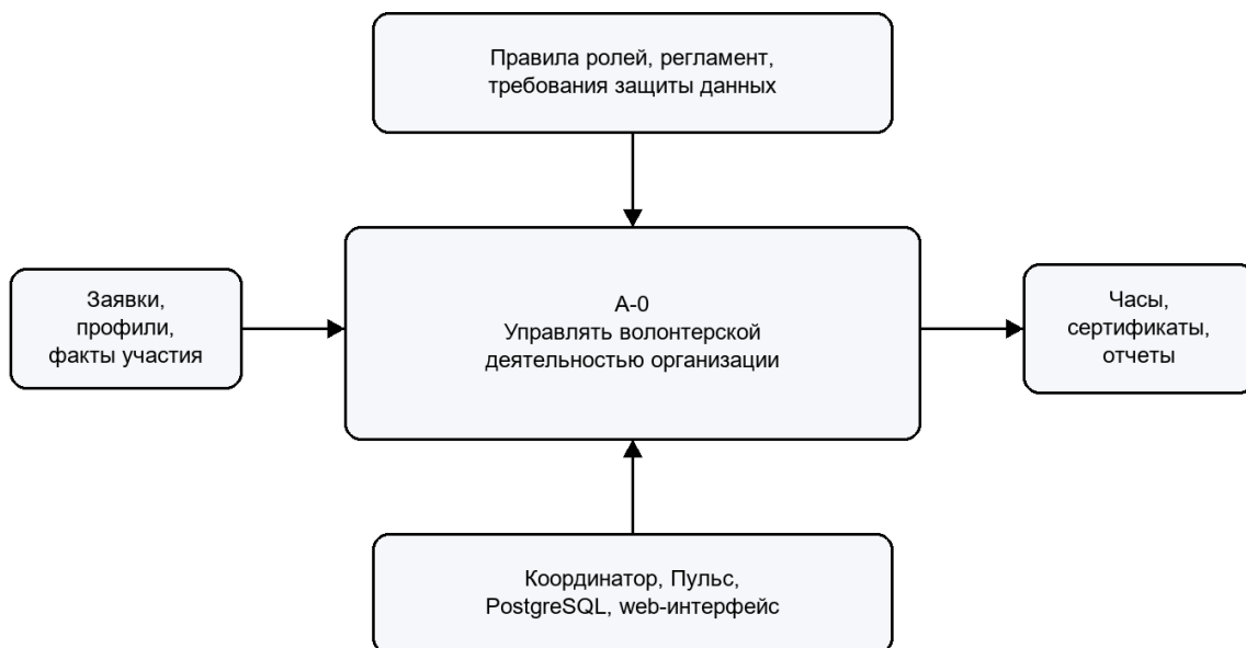
Рисунок 2 - Контекстная диаграмма IDEF0 управления волонтерской деятельностью
