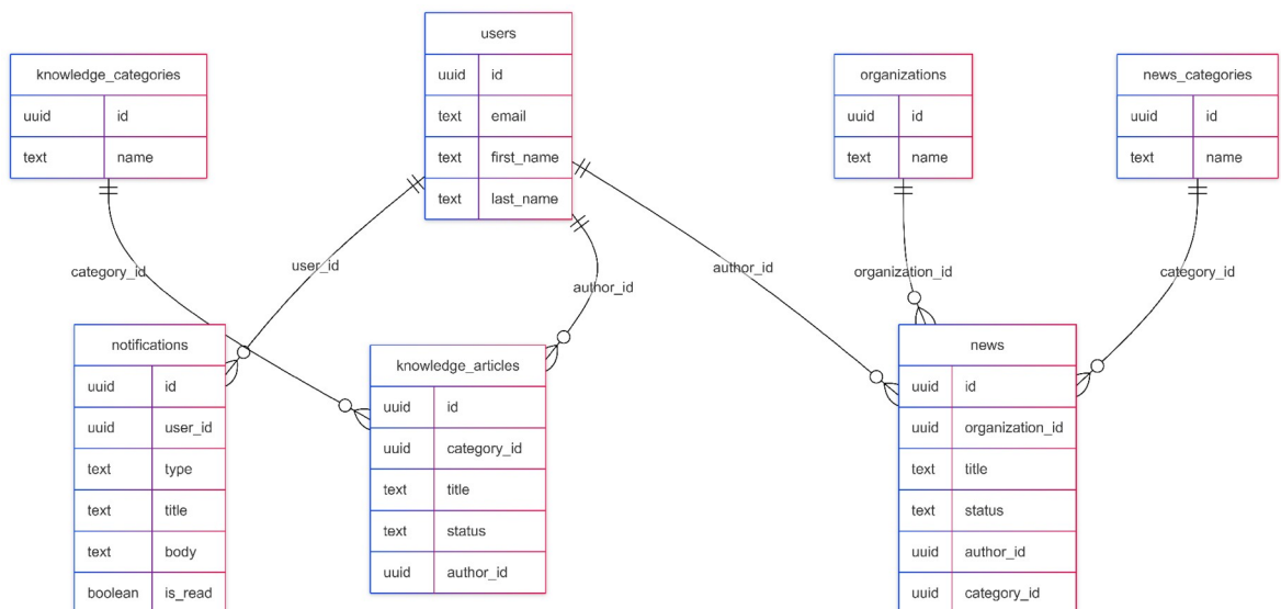
Рисунок 17 - ER-диаграмма подсистемы контента и уведомлений
