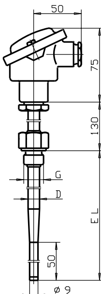
型号 902002/11
