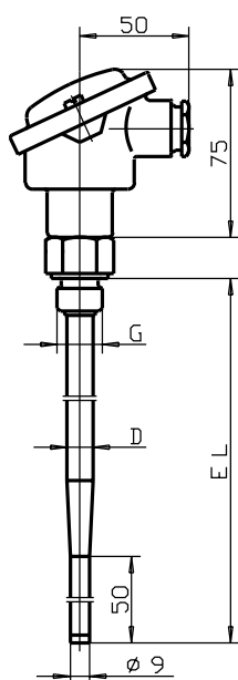
型号 902002/21
