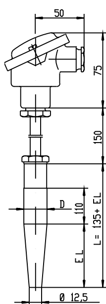
型号 902002/51
