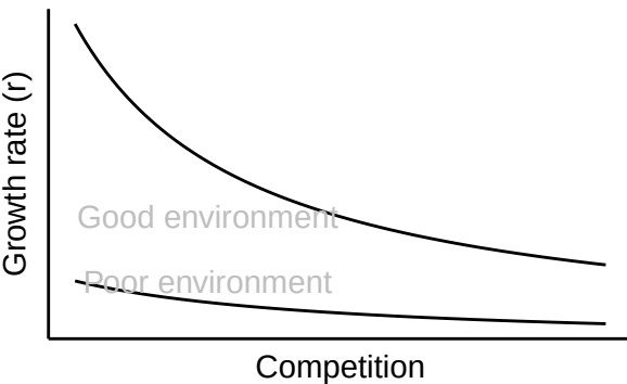
Subadditive
