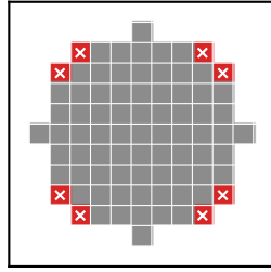
(a) \text{disk}(5) \circ \text{disk}(4) \neq \text{disk}(5)
