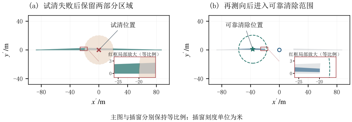
图 7 实际试清失败与后续定位。主图保持等比例，插窗为明确标注的局部放大。蓝色表示观测位置域，绿色表示试清失败后保留部分，灰色为后续测向前区域；圆圈分别为 20 米试清和 19.5 米可靠清除范围。局部坐标仅由平移、旋转得到，未使用真实源坐标。
