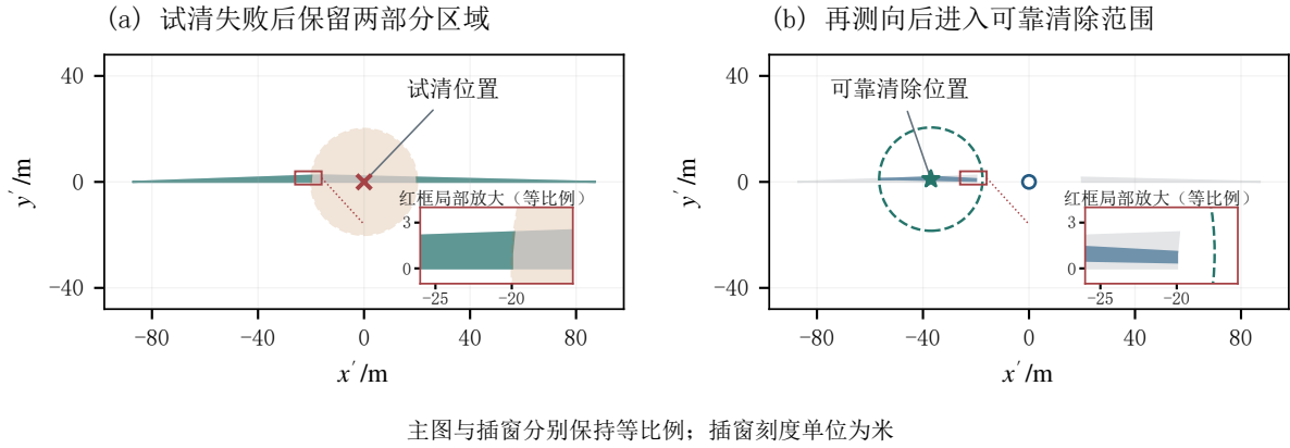
图 8 实际试清失败与后续定位。主图保持等比例，插窗为明确标注的局部放大。蓝色表示观测位置域，绿色表示试清失败后保留部分，灰色为后续测向前区域；圆圈分别为 20 米试清和 19.5 米可靠清除范围。局部坐标仅由平移、旋转得到，未使用真实源坐标。
