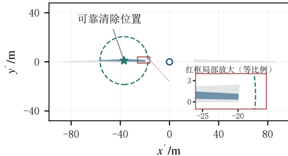
(b) 再测向后进入可靠清除范围
