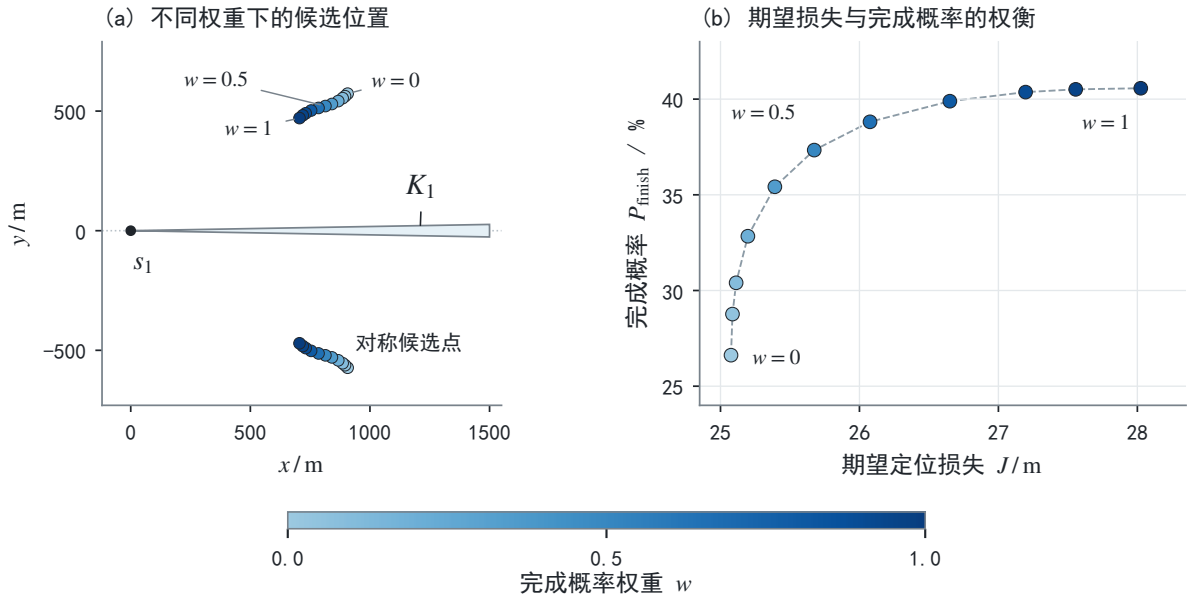
图 3 11 个权重下的候选检测点及评价指标 ( a = 0, \beta = 0 )。颜色表示完成概率权重，虚线仅连接相邻权重的数值结果，不表示点间所有位置都已入选。
