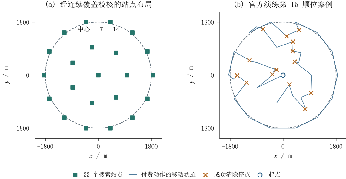
图 7 固定搜索布局与一次完整执行轨迹。右图取 M32 的 30 场官方演练中按单场秒/源排序的第 15 场，结果为 445.24 s/源；连线由已接受的付费动作位置重建。叉号表示成功清除时的机器人停点，不表示源的真实坐标。
