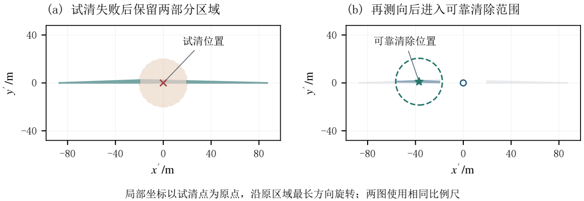
图 3 同一官方演练中频道 3 的试清与后续定位。图 (a) 蓝色为试清前区域，绿色为失败后保留部分，橙色圆为 20 米试清范围；图 (b) 灰色为失败后区域，蓝色为再测向后的区域，虚线圆为 19.5 米安全清除范围。局部坐标 x', y' 由原坐标平移、旋转得到，图形未使用真实源坐标。
