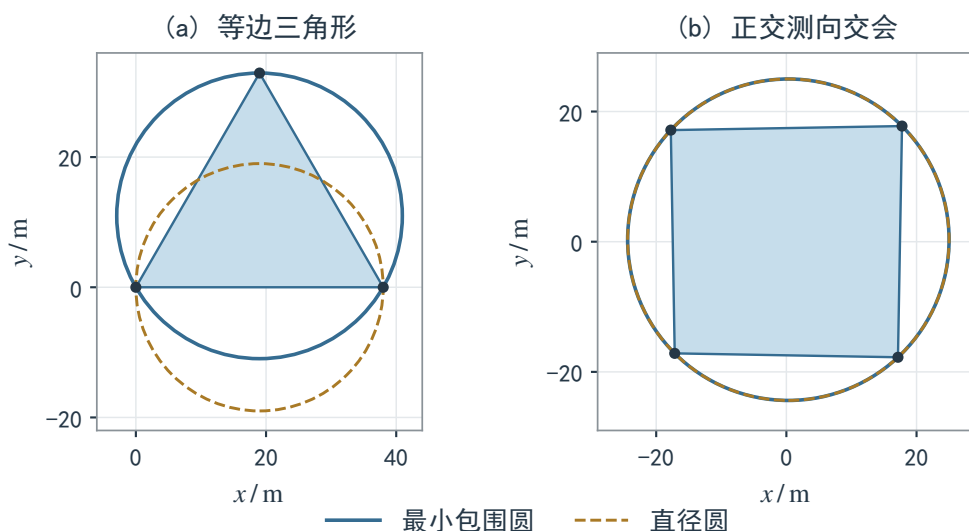
图 2 两类交会区域的覆盖结果。左：边长 38 米的等边三角形，其直径圆不能覆盖整个区域；右：两次正交示向度形成的四边形，其直径圆能够覆盖整个区域
