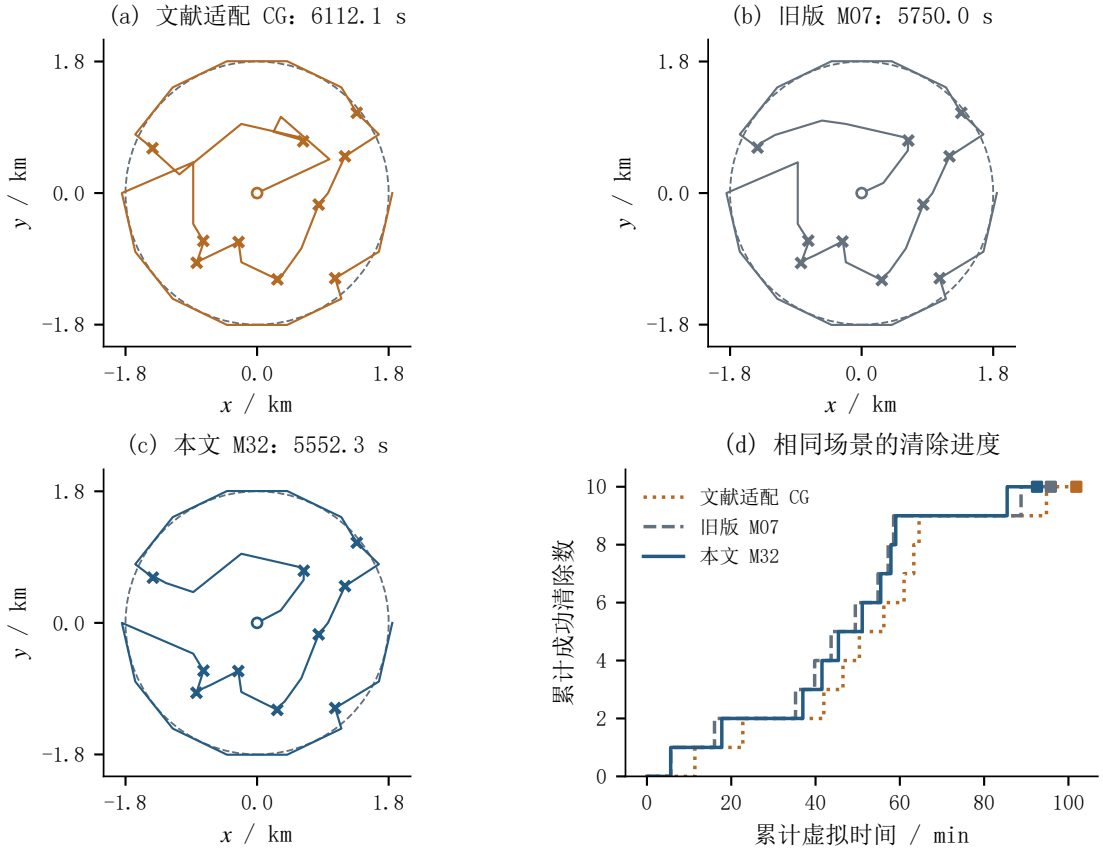
图 13 三策略在同一场景的路径与清除进度。取全部 30 个本地场景按 M07 减 M32 的秒/源差值排序第 15 场，含 10 源、其中 3 个定向；圈为起点，叉为成功清除停点，非源真值。坐标等比例且范围相同；进度曲线延续至搜索完成，末端方块表示任务结束，时间计入全部付费动作。
