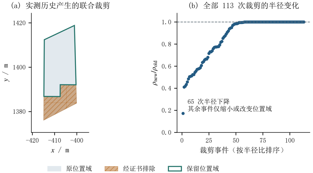
图 11 联合约束如何促成可靠清除。左图取全部 65 次半径严格下降事件按相对降幅排序的第 33 次，橙色斜线区为排除部分；右图展示 M32 30 场官方演练的全部 113 次裁剪，65 次降低包围圆半径，半径比中位数为 0.9972。事件非独立场景，不将 113 当作性能样本量。
