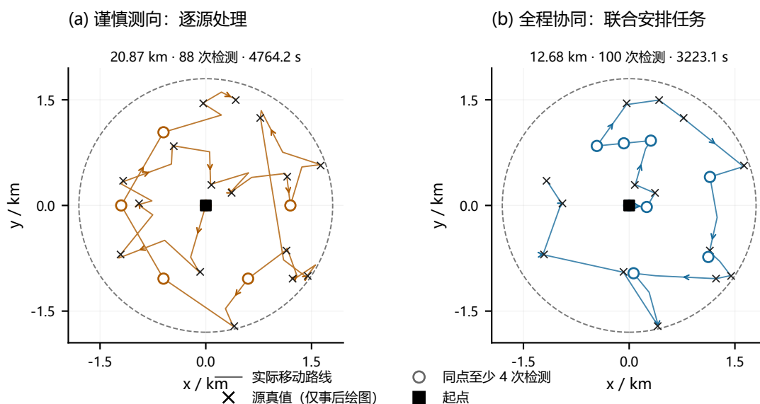
同场景本地对照 · 种子 2026092410 · 16 个源
