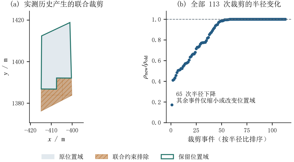
图 2 联合约束如何促成可靠清除。左图取全部 65 次半径严格下降事件按相对降幅排序的第 33 次，橙色斜线区为排除部分；右图展示联合域规划 30 场官方演练的全部 113 次裁剪，65 次降低包围圆半径，半径比中位数为 0.9972。事件非独立场景，不将 113 当作性能样本量。
