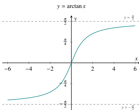
图 5: 反正切函数 y = \arctan x
