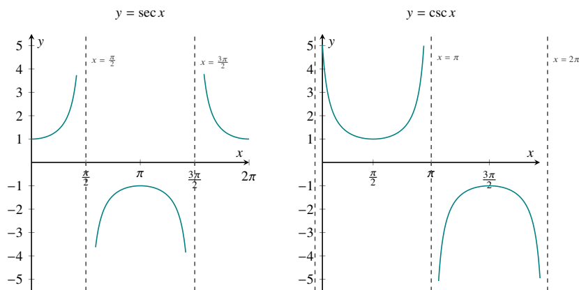
图 2: 正割函数 y = \sec x 与余割函数 y = \csc x
