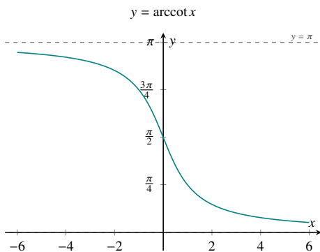
图 6: 反余切函数 y = \operatorname{arccot} x
