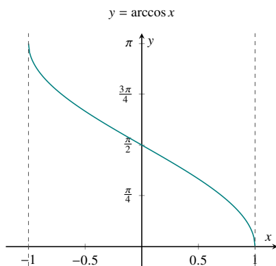
图 4: 反余弦函数 y = \arccos x
