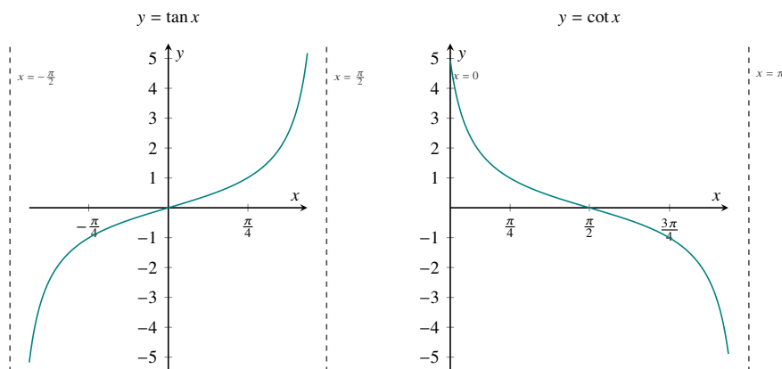
图 1: 正切函数 y = \tan x 与余切函数 y = \cot x
