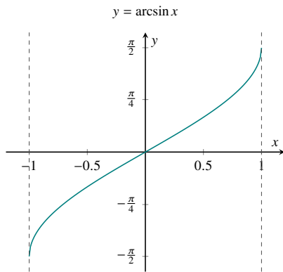
图 3: 反正弦函数 y = \arcsin x
