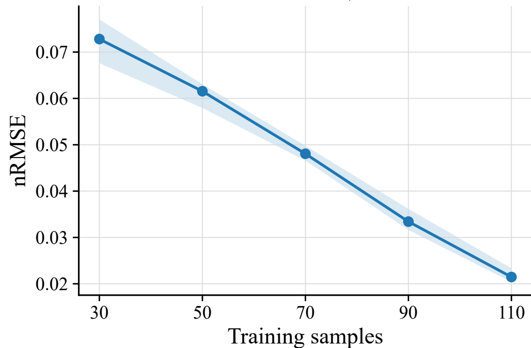
nRMSE ↓
