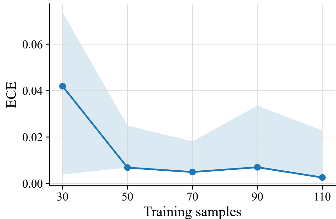
ECE ↓
