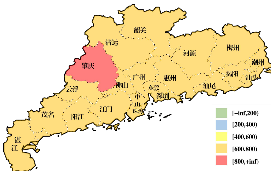
图 2-1 运行日 2026-1-9 统调负荷高峰时刻日前节点电价分布图
