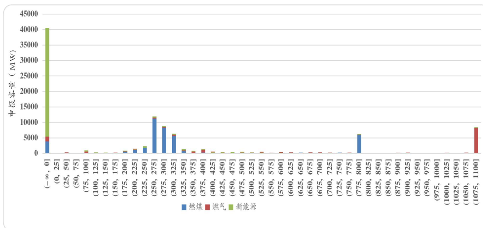
图 1 运行日 2026-1-9 日报价分布（不含检修和低于最小技术出力的容量）
