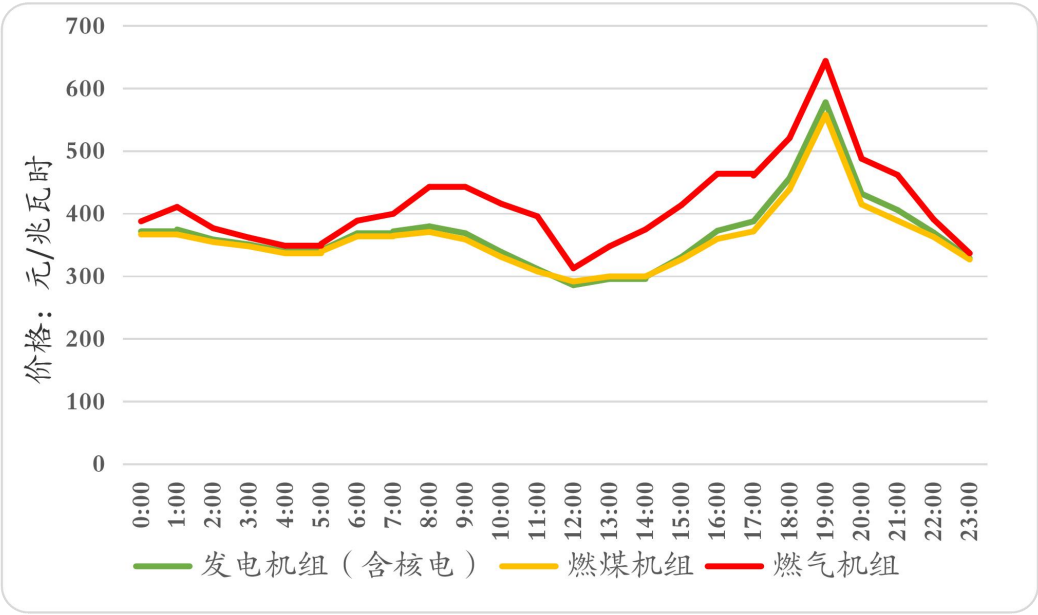
图 4 运行日 2026-3-25 日全省发电侧加权价格曲线
