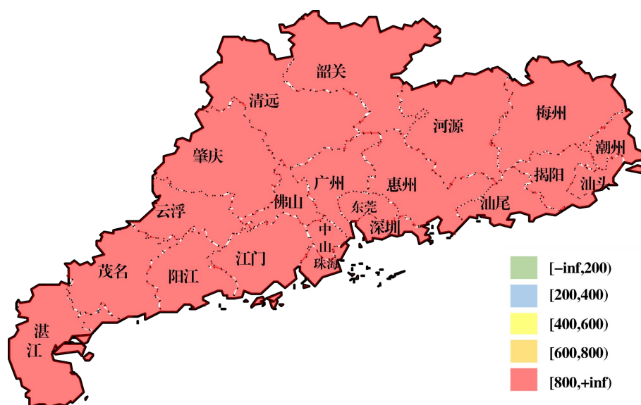
图 2-1 运行日 2026-3-25 统调负荷高峰时刻日前节点电价分布图
